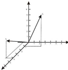
Gambar 3. Plot data matriks \mathbf{X} untuk n = 3 pada p = 2
