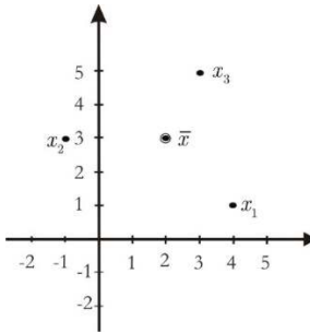
Gambar 2. Plot data matriks \mathbf{X} untuk n = 3 pada p = 2
