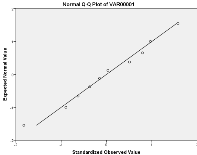
Gambar 4. Normal Q-Q Plot nilai Ekspektasi v.s Nilai Pengamatan Terstandar
