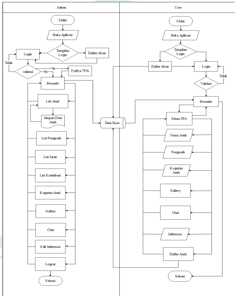
Gambar IV. 2. Flowmap sistem yang diusulkan
