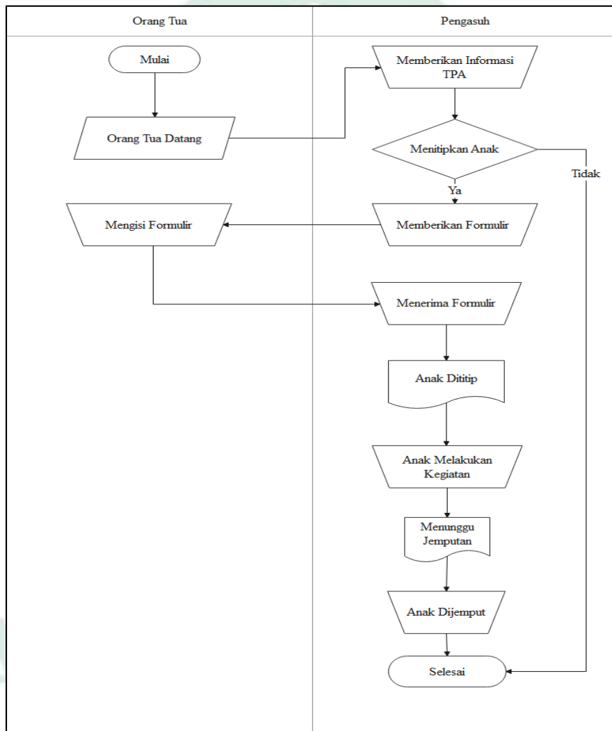
Gambar IV. 1. Flowmap sistem yang sedang berjalan
