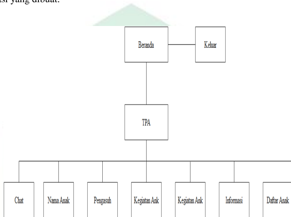
Gambar IV. 11. Struktur Navigasi
