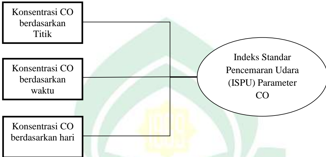
Gambar 2.2 Kerangka Konsep
