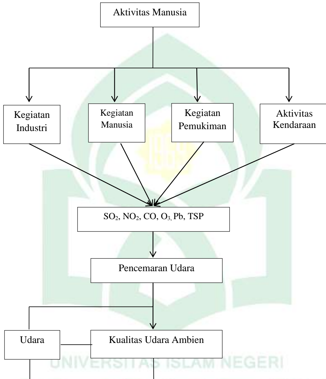
Gambar 2.1 Kerangka Teori
