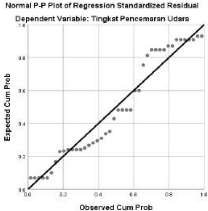
Gambar 4.4 Hasil Uji Normalitas Sore
