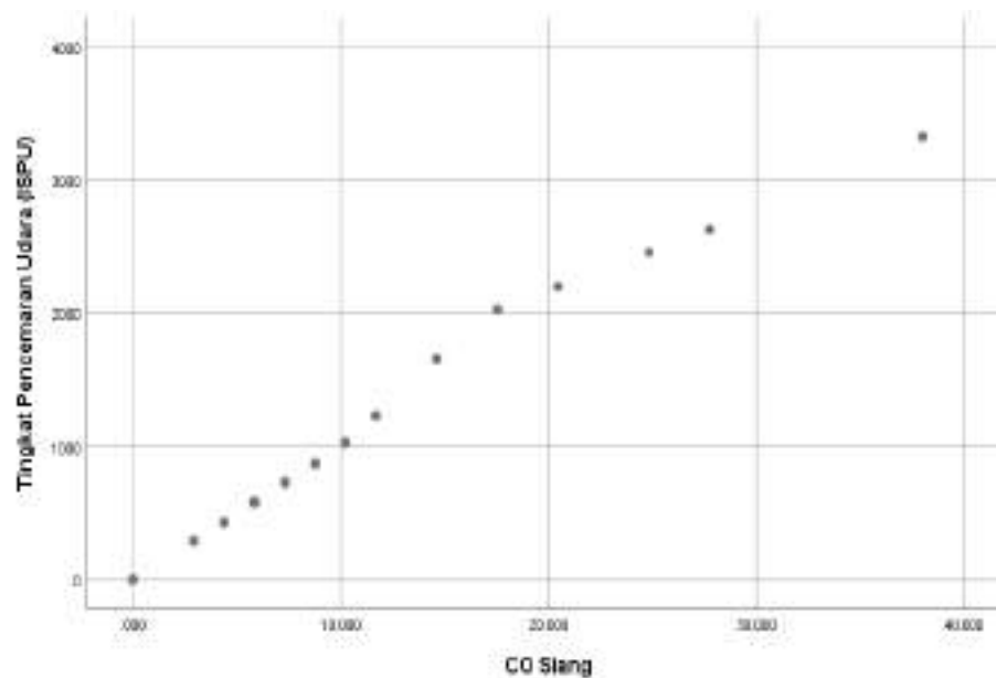
Gambar 4.9 CO mempengaruhi tingkat pencemaran udara (ISPU)
