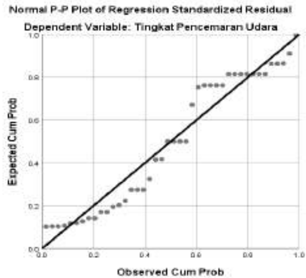
Gambar 4.2 Hasil Uji Normalitas Data Pagi
