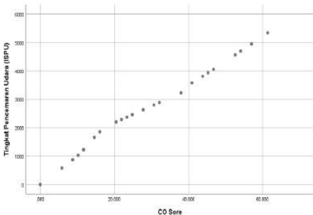
Gambar 4.10 CO mempengaruhi tingkat pencemaran udara (ISPU)
