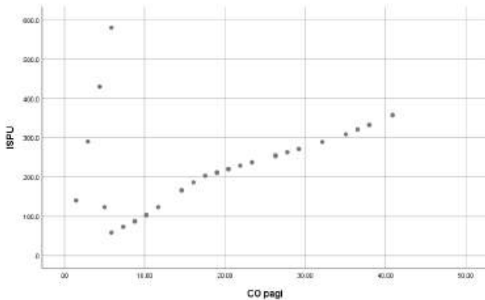
Gambar 4.8 CO mempengaruhi tingkat pencemaran udara (ISPU)
