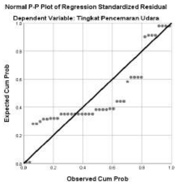
Gambar 4.3 Hasil Uji Normalitas Data Siang
