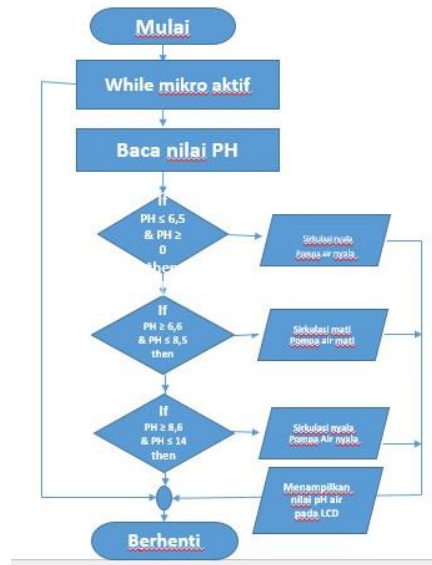
Gambar IV.4. Rangkaian Flowchart Sistem Sirkulasi dan Pengukuran pH Air pada Tambak Udang Berbasis Arduino 3. Perancangan Perangkat Keras
