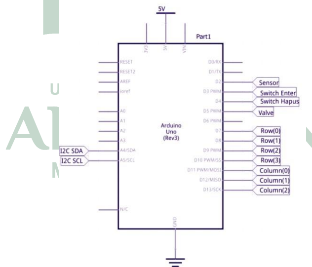
Gambar IV.5 Rangkaian Arduino Uno (Djuandi, 2011)
