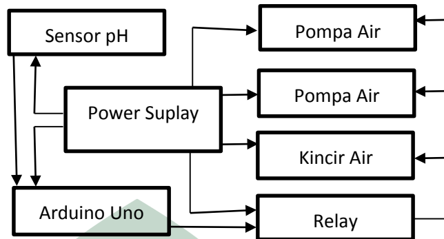
Gambar IV.3. Diagram Blok alat sirkulasi dan pengukuran Ph air pada tambak berbasis Arduino terdiri dari beberapa masukan dan keluaran.
