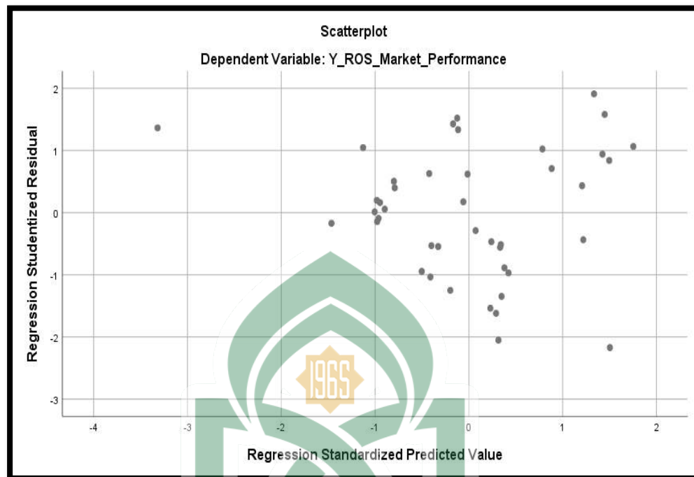
Gambar 4.3 Grafik Scatterplot
