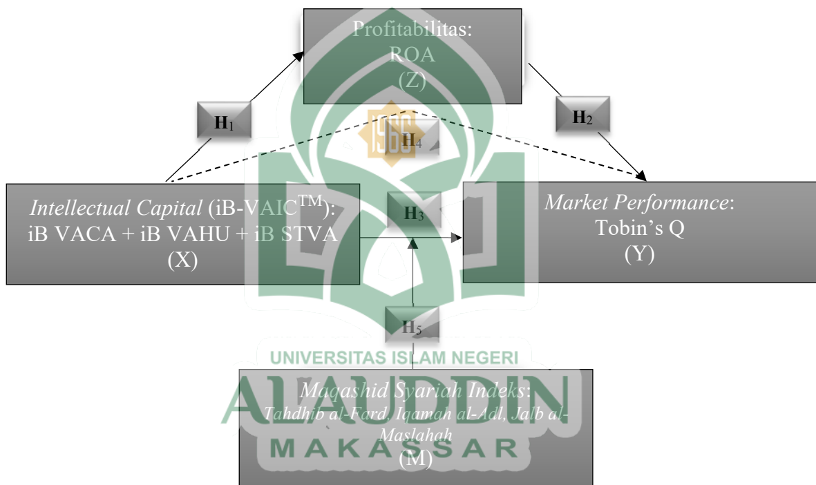
Gambar 2.2 Kerangka Pikir
