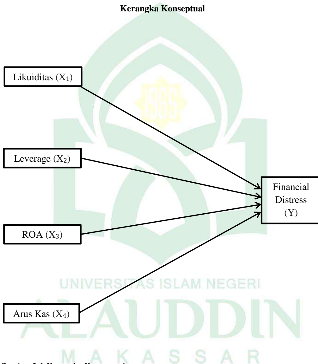
Gambar 2.1 Kerangka Konseptual
