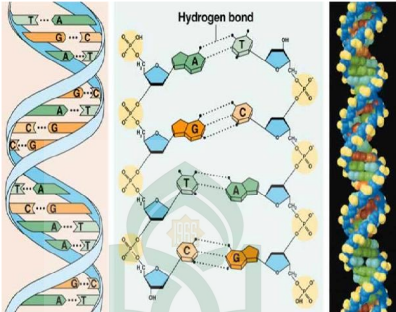
Gambar 2.5. Struktur double heliks DNA
