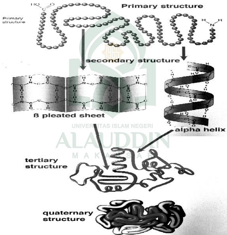
Gambar 2.8. Tingkatan struktur protein
