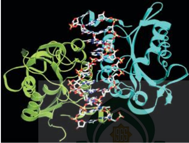
Gambar 3.1 Struktur enzim restriksi Bam HI yang mengikat DNA. Enzim tersebut mengenali double strand dari DNA dengan dengan sekuens spesifik 5'-GGATCC-3', yang selanjutnya memecah ikatan fosfodiester antara dua residu G. Hasilnya adalah berupa dua fragmen yang ujungnya sticky ends . Pada gambar tersebut warna hijau dan biru menunjukkan subunit protein dimer yang identik (Reece, 2007).
