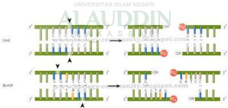
Gambar 3.2 Contoh pola pemotongan enzim restriksi endonuklease. Enzim tersebut menghidrolisis ikatan fosfodiester yang menghasilkan formasi 5'-PO 4 - dan 3'-OH yang bagian terminalnya berbentuk asimetris atau sticky ends ( Bam HI) dan bentuk simetris atau blunt ends ( Sma I) (Allison, 2007).
