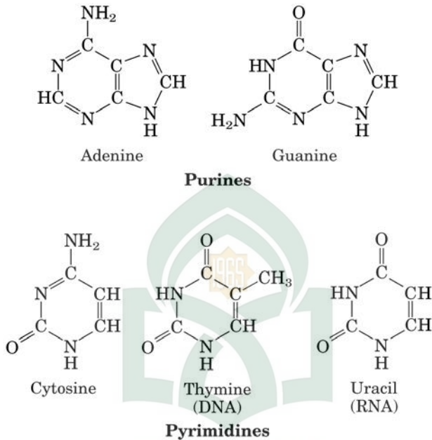
Gambar 2.3. Struktur Purin dan Pyrimidin (Adenin dan Guanin; Cytosin, Tymin dan Urasil)
