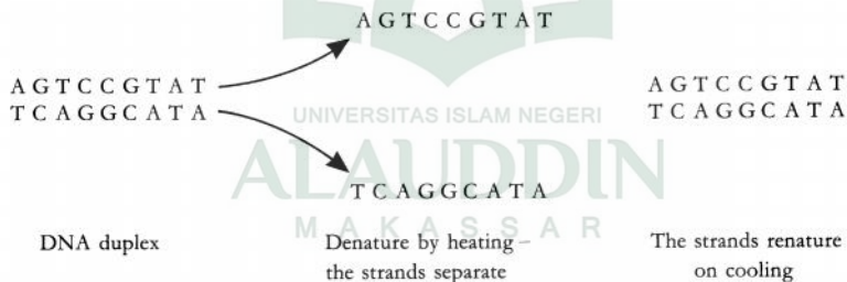
Gambar 6.1 Prinsip Dasar hibridisasi koloni
