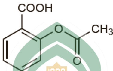
Gambar 1. Struktur Aspirin (Sweetman, 2009: 20)
