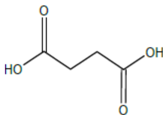
Gambar 5. Struktur Asam Suksinat (O'Neil et al. 2001)
