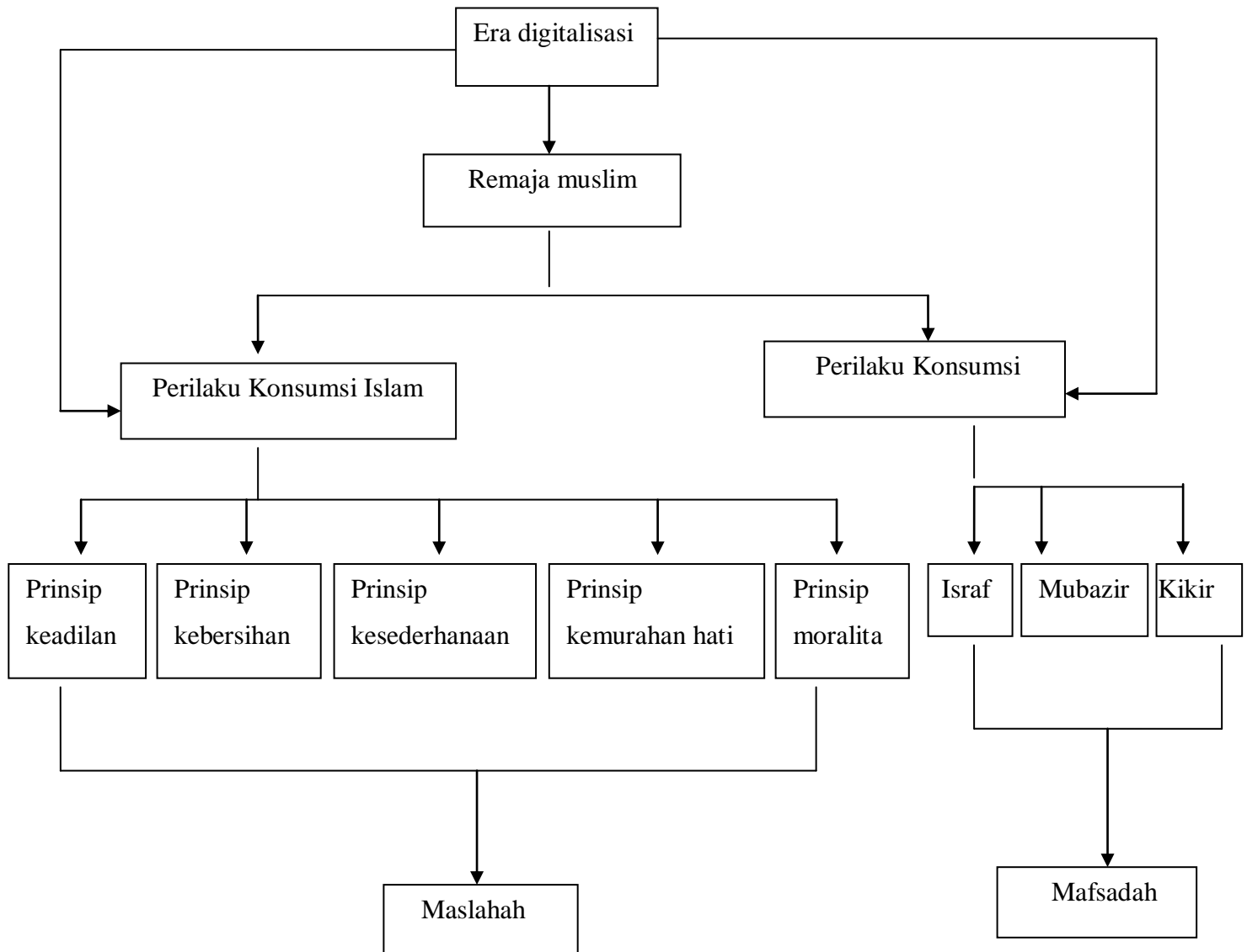
Gambar 2.1 Kerangka Berpikir
