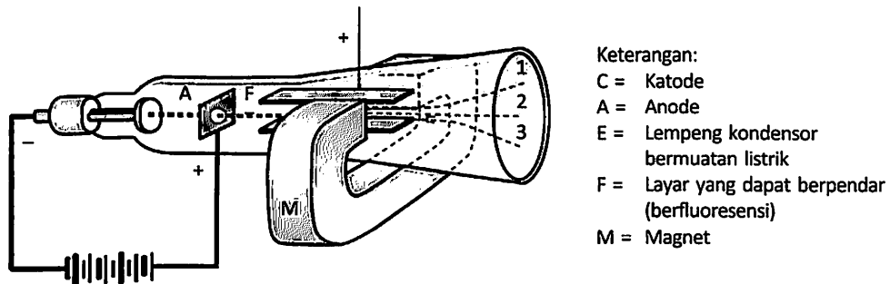
Gambar 3.1. Skema pembentukan sinar katoda
