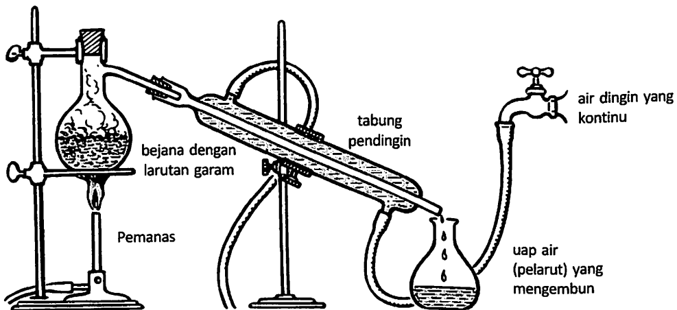
Gambar 6.5 Pemisahan campuran dengan proses distilasi
