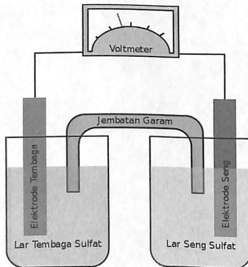
Gambar 8.5 Larutan elektrolit dalam sebuah baterai
