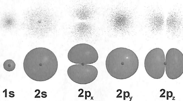
Gambar 3.2 Orbital elektron
