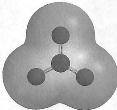
Gambar 8.4 Medan potensial elektrostatik dari ion Nitrat ( \text{NO}_3^- )
