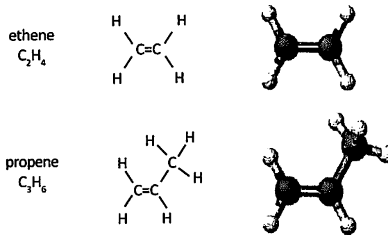
Gambar 5.2 Rantai ethena dan propena
