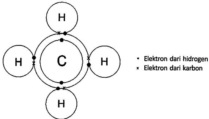
Gambar 8.2 Molekul metana
