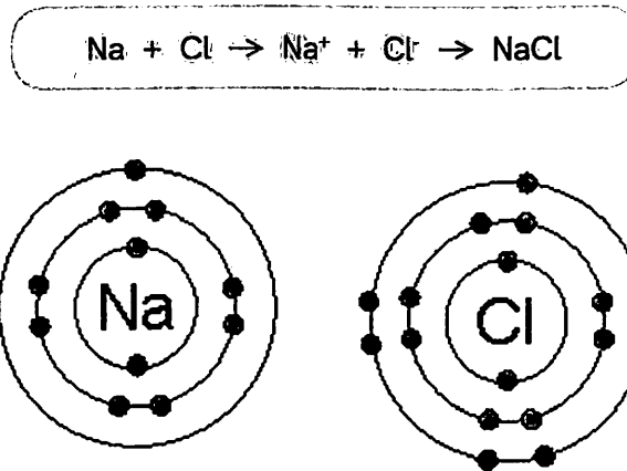
Gambar 8.3 Ikatan natrium dan klor membentuk Natrium Klorida
