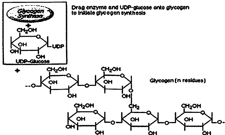
Gambar 12.3 Sintesis Glikogen
