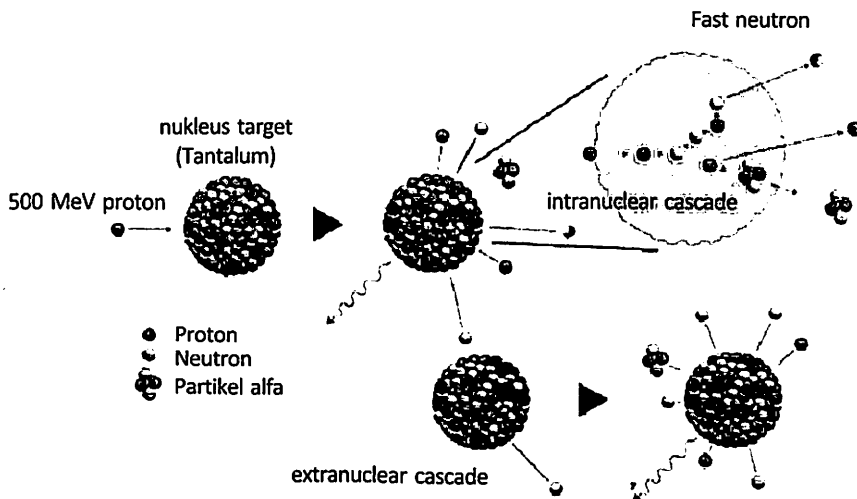
Gambar 3.6 Proses Spallasi
