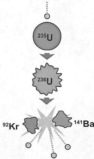
Gambar 3.5 Reaksi fisi nuklir
