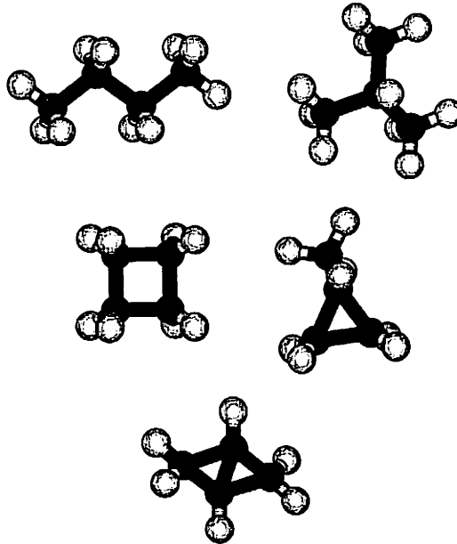
Gambar 5.1 Contoh rantai beberapa hidrokarbon alifatik
