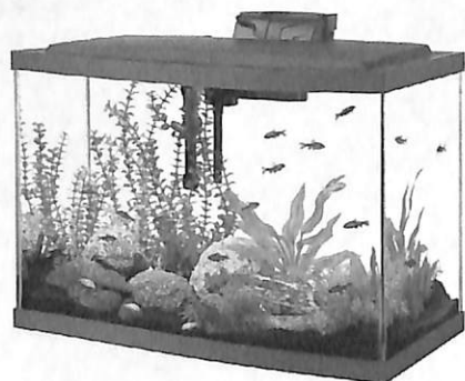
Gambar 8.6 Analogi asam basa dengan keadaan lingkungan di akuarium
