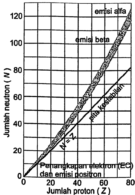
Gambar 3.6 Grafik pita kestabilan inti atom
