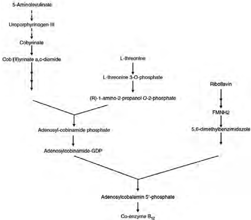
Gambar 3.1 Intermediet utama dari sintesis biologis cobalamin. Panah dengan garis tidak lengkap menunjukkan adanya lebih dari tiga langkah enzimatik yang terlibat dalam memperoleh zat antara (LeBlanc et al., 2016).
