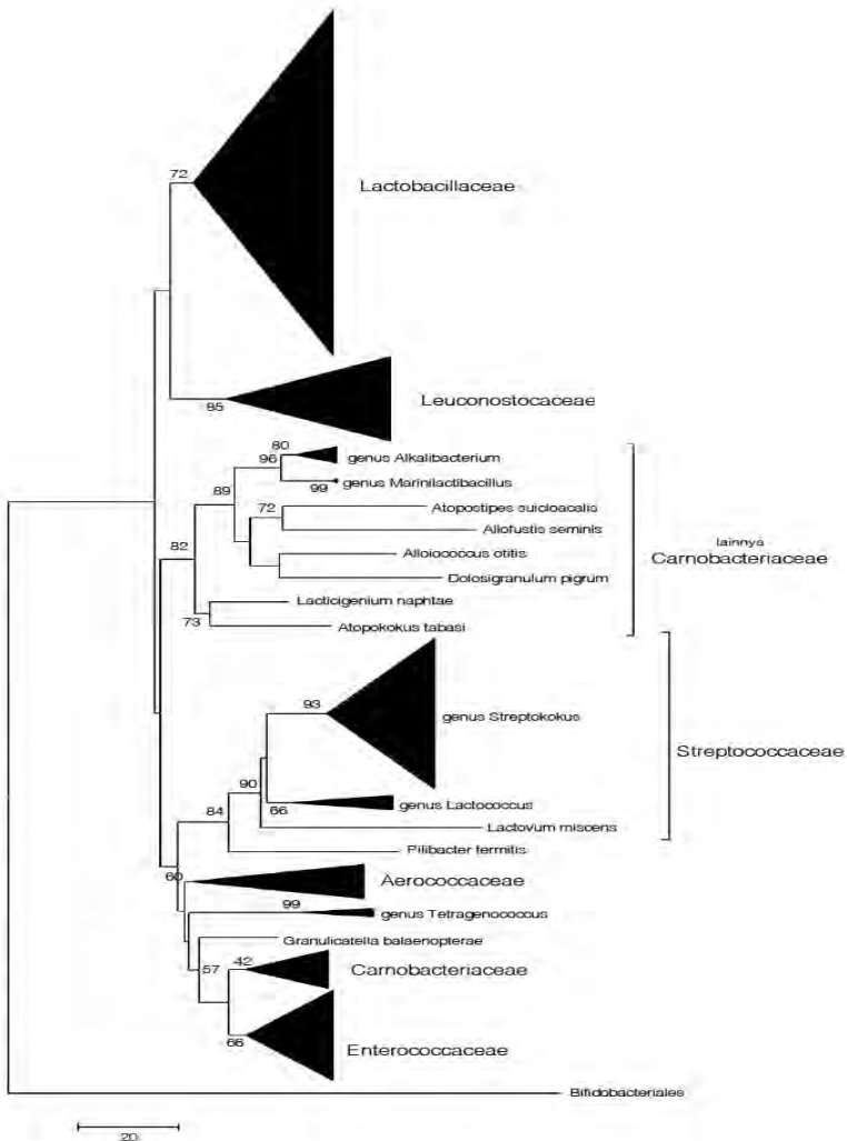
Gambar 1.1 Pohon filogenetik hubungan antarfamili pada ordo Lactobacillales berdasarkan urutan gen 16S rRNA menggunakan Neighbor-Joining . Nilai bootstrap (1.000 ulangan). Bilah skala mewakili jumlah substitusi per situs (Felis et al., 2016).
