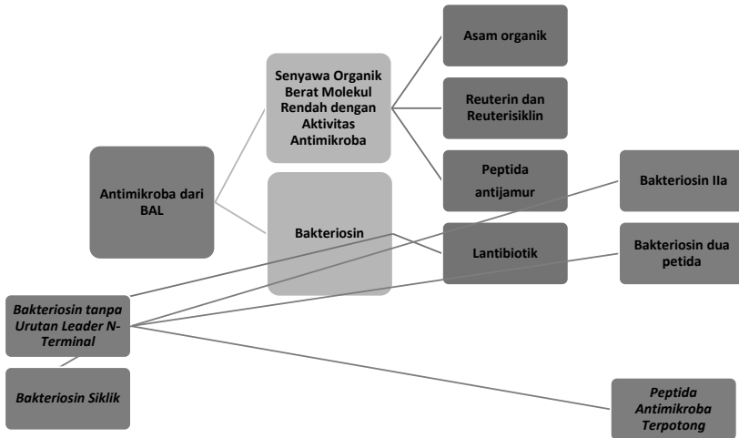
Gambar 2.1 Kelompok Senyawa antimikroba yang Dihasilkan oleh BAL
