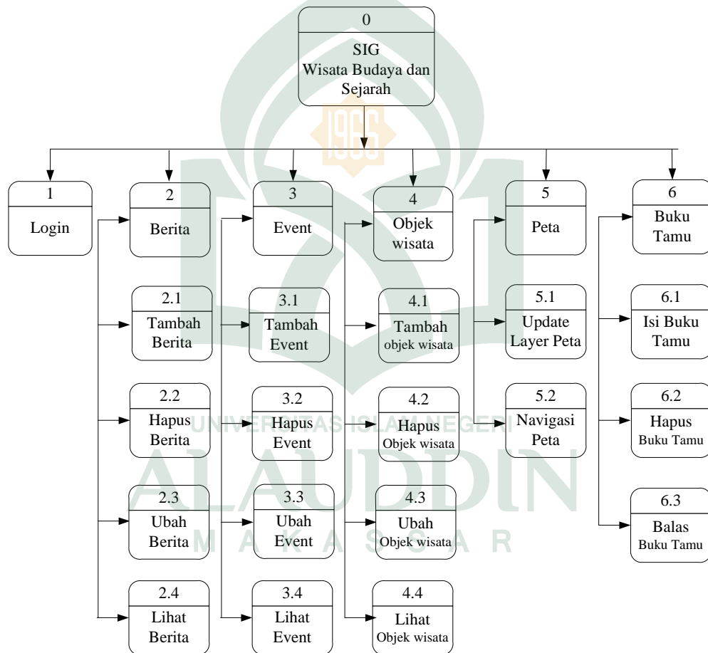
Gambar 4.3 Diagram Berjenjang
