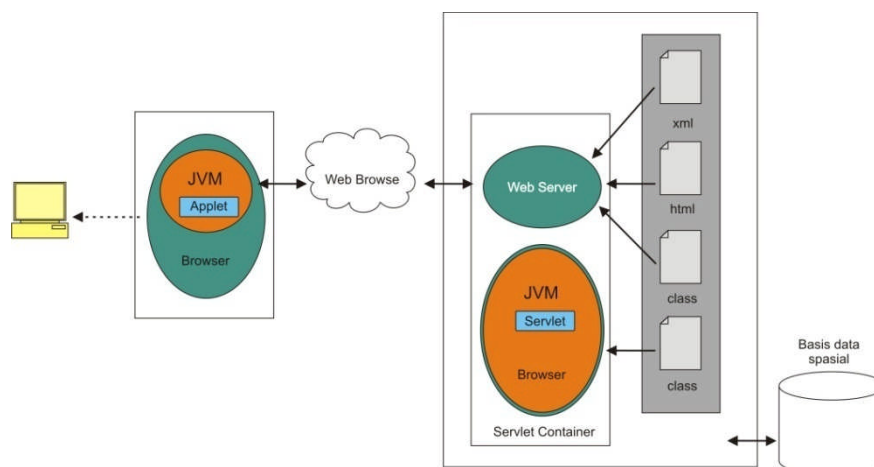
Gambar 2.6 Komunikasi Applet dan Servlet menggunakan ALOV Map (Sumber : http://ilmutanahuns.files.wordpress.com )
