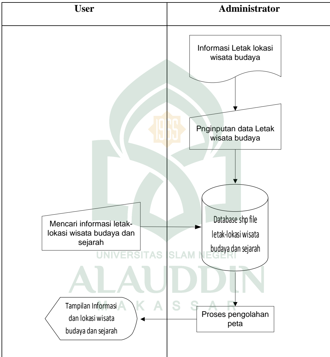
Gambar 4.2 Bagan Alir Sistem yang diusulkan
