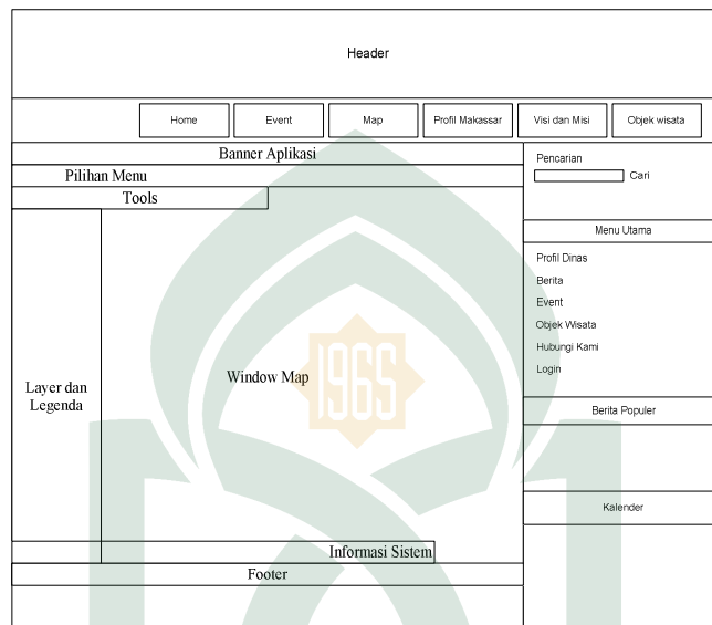
Gambar 4.13 Rancangan Output Map
