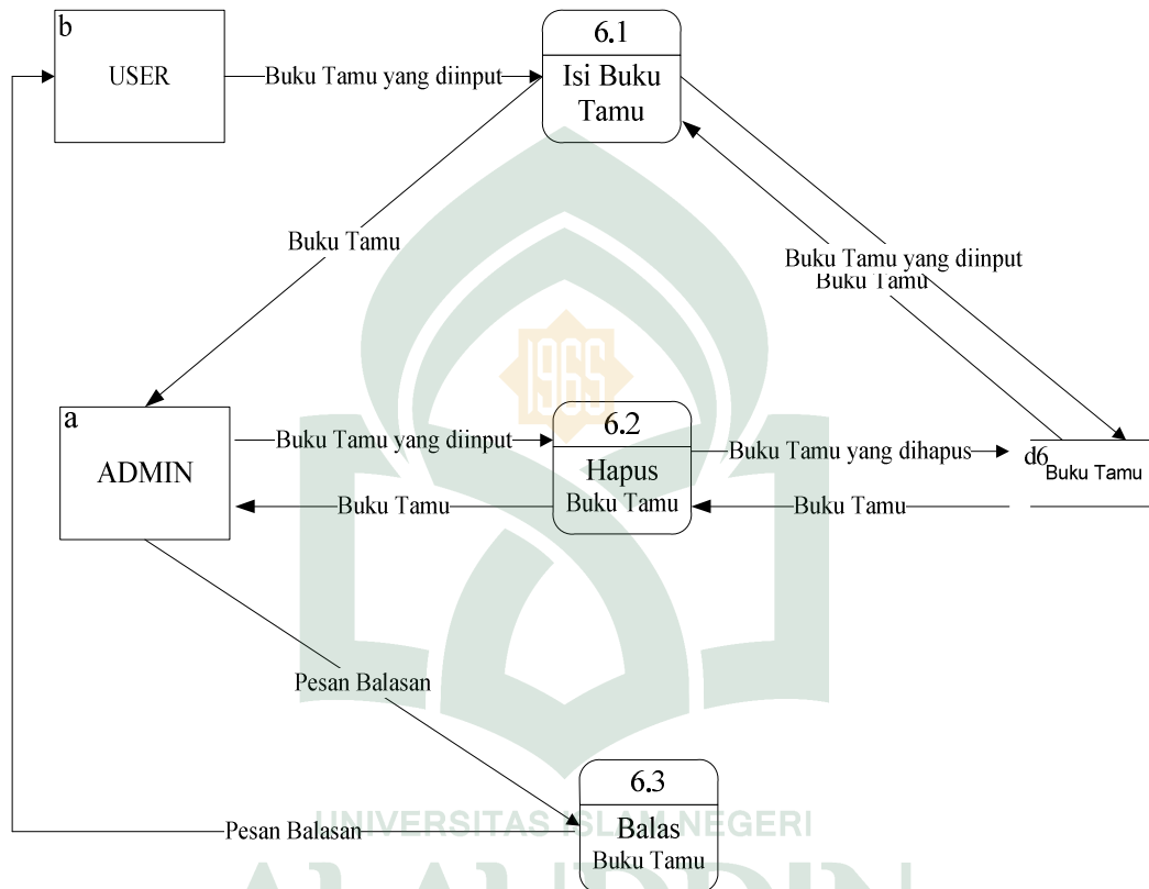
Gambar 4.10 DFD level 1 Proses Buku Tamu
