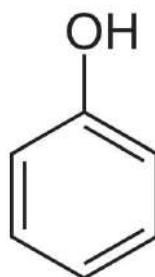
Gambar II. 4 Struktur Fenol (Kusnadi, 2018)
