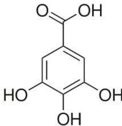
Gambar II. 5 Struktur Asam Galat (Junaidi & Anwar, 2018)
