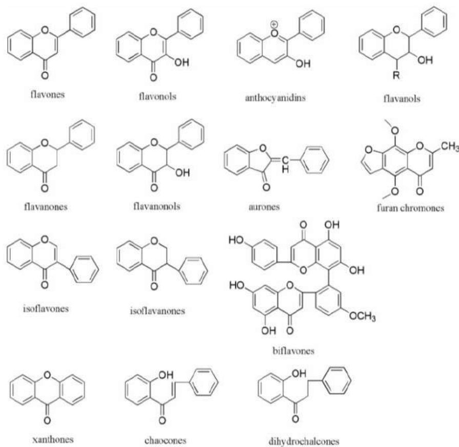
Gambar II. 3 Struktur Kimia Dan Klasifikasi Flavonoid (Tian Yang Wang et al, 2018)
