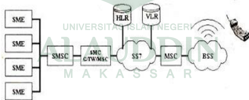
Gambar II.2 Arsitektur jaringan SMS (Riadi, 2016).
