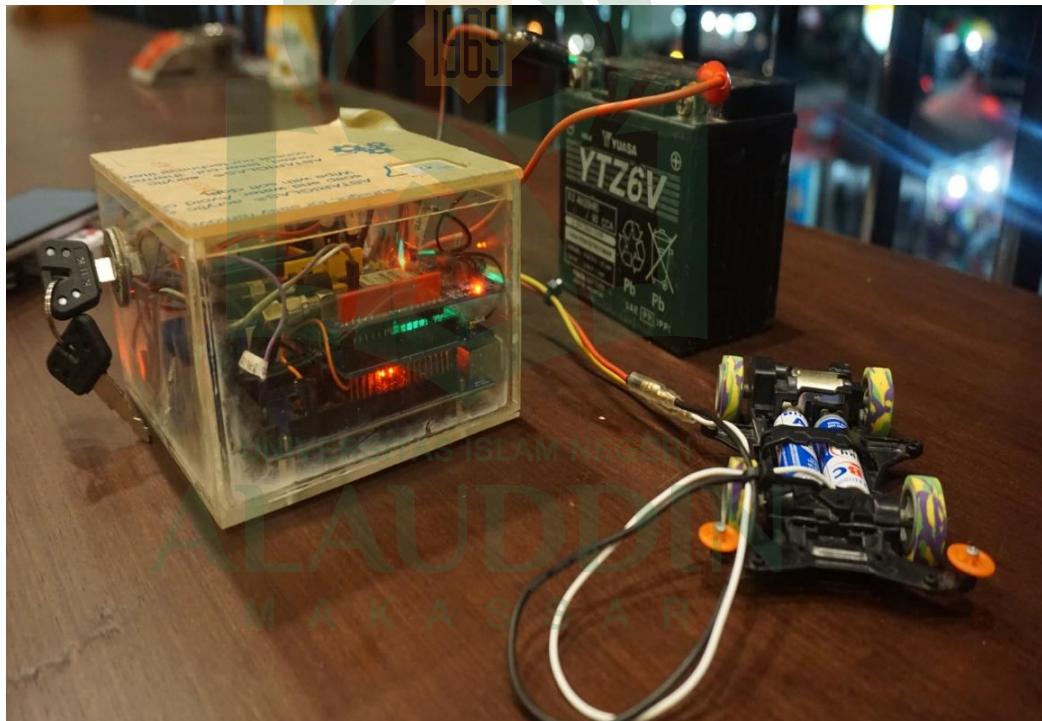
Gambar V.1 Hasil Rancangan Alat secara keseluruhan dalam keadaan tertutup
