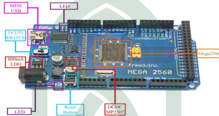
Gambar II.3 Arduino Mega 2560 (Oktariawan, 2015).
