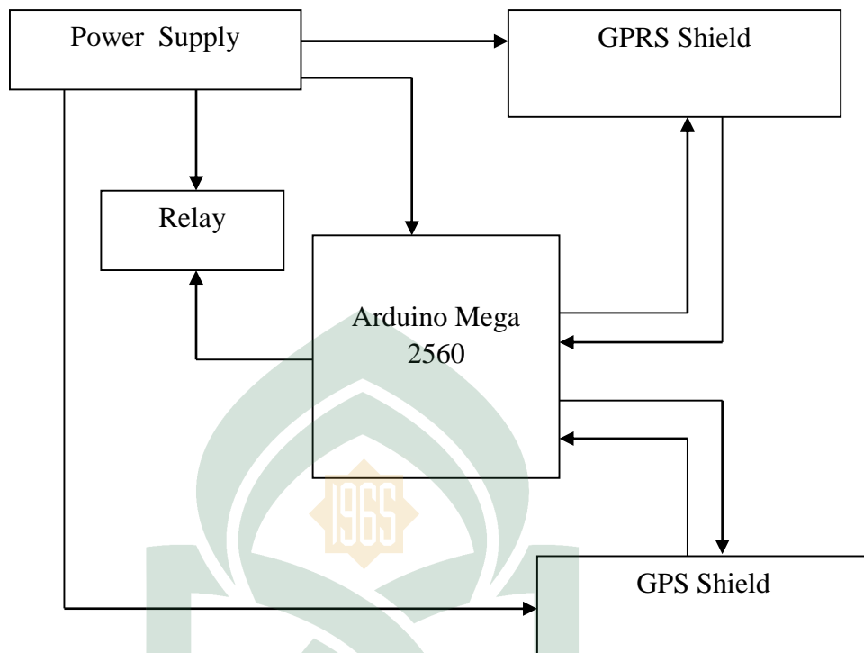
Gambar IV.1 Diagram Blok Sistem Keamanan Kendaraan Bermotor Menggunakan SMS Dengan Metode GPS Tracking Berbasis Arduino terdiri dari beberapa masukan dan keluaran.
