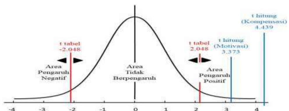
Kurva Uji t (Parsial)
