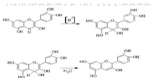
Gambar 3. Reaksi Identifikasi Flavonoid
