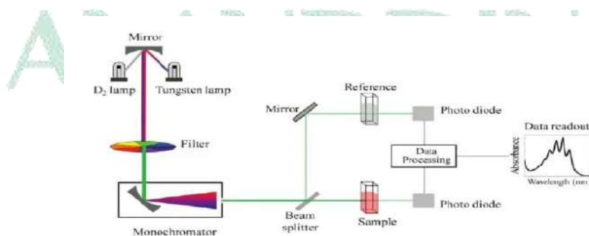
Gambar 2. Skema Kerja Spektrofotometer UV-Vis Jenis Double-Beam
