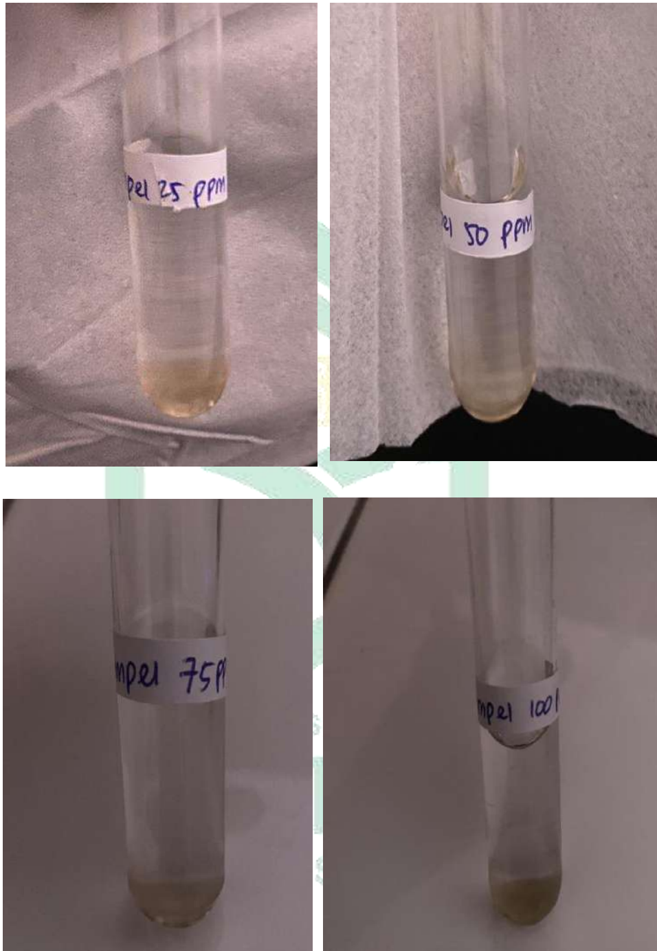
Sampel + Asetat Anhidrat + Asam Sulfat
