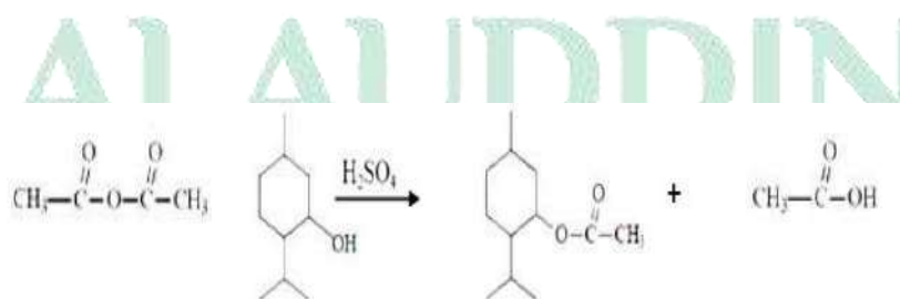
Gambar 5. Reaksi Identifikasi Steroid/Terpenoid
