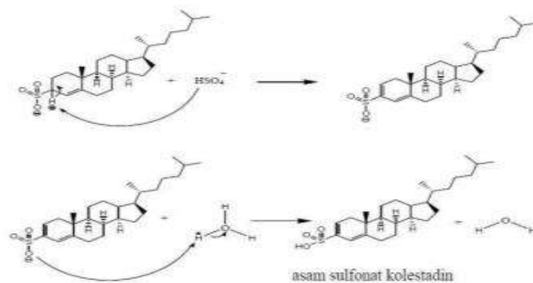
Gambar 6. Ikatan Kimia Antara Flavonoid Dan Kolesterol (Moelok, 2006)
