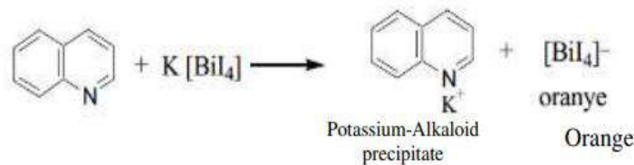
Gambar 4. Reaksi Identifikasi Alkaloid
