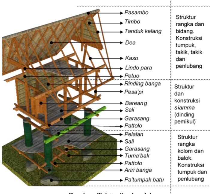
Gambar: Tektonika Landa'
