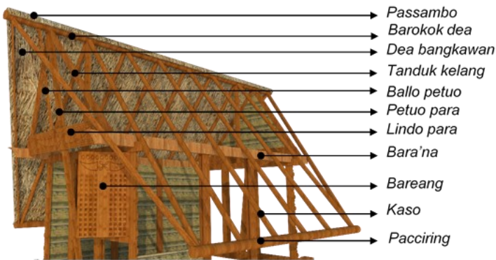
Gambar: Struktur dan konstruksi atap Landa'
