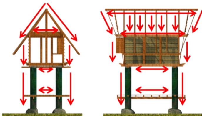
Gambar: Ilustrasi Pembebanan Landa'
