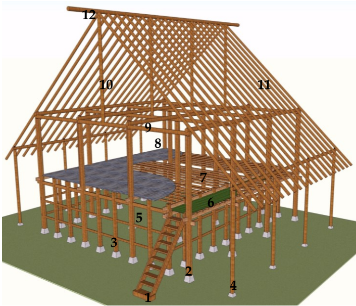
Gambar. Struktur dan Konstruksi
