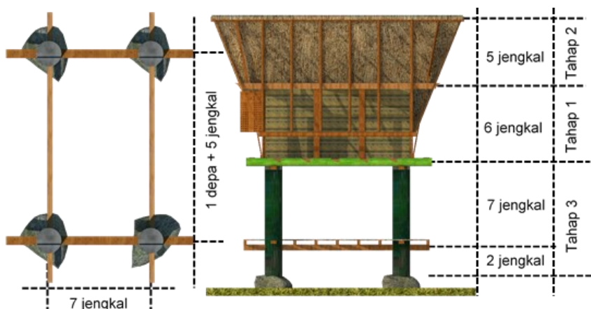
Gambar: Ukuran denah dan tinggi dari Landa'
