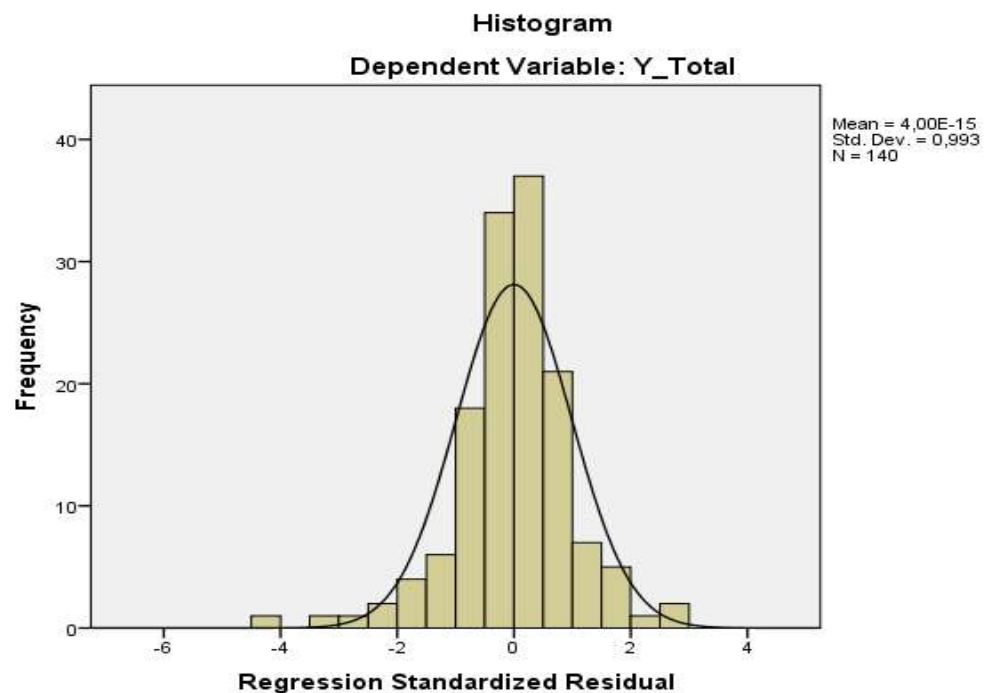
Gambar 4.1 Metode Grafik Histogram
