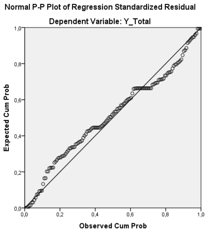
Gambar 4.2 Metode Grafik Normal P-Plot
