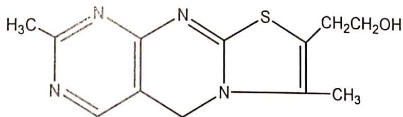
Gambar 10.2. Tiokrom
