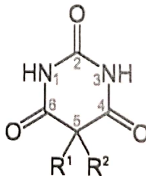
Gambar 7.2. Struktur Barbiturat
