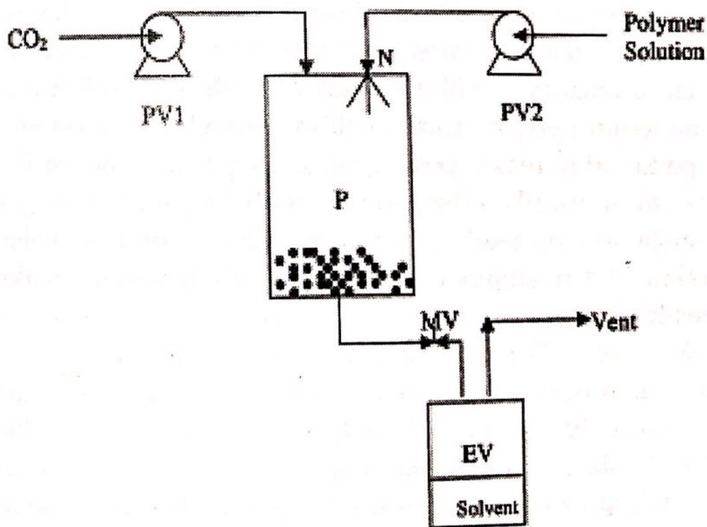
Gambar 20. Diagram skematik metode SAS: PV1 dan PV2 adalah dua pompa volumetric, N adalah nosel
