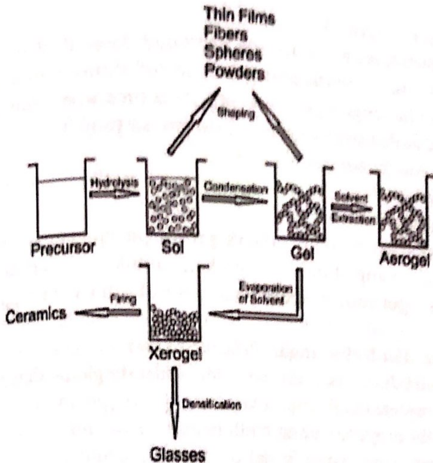
Gambar 11. Tahapan preparasi dengan metoda sol gel
