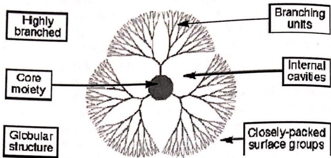
Gambar 4. Gambaran skematik dendrimer, memperlihatkan inti, cabang, dan permukaan
