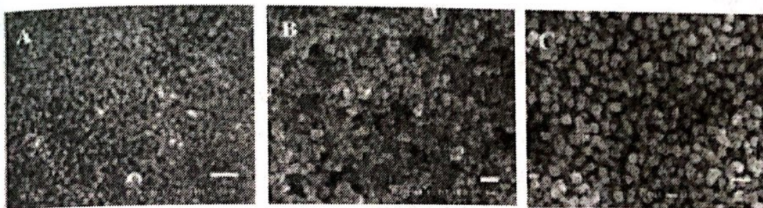
Gambar 15. Gambar FESEM dari nanopartikel quasi sferikal perilen dengan berbagai macam ukuran (a) 25 nm, (b) 60 nm, dan (c) 90 nm.
