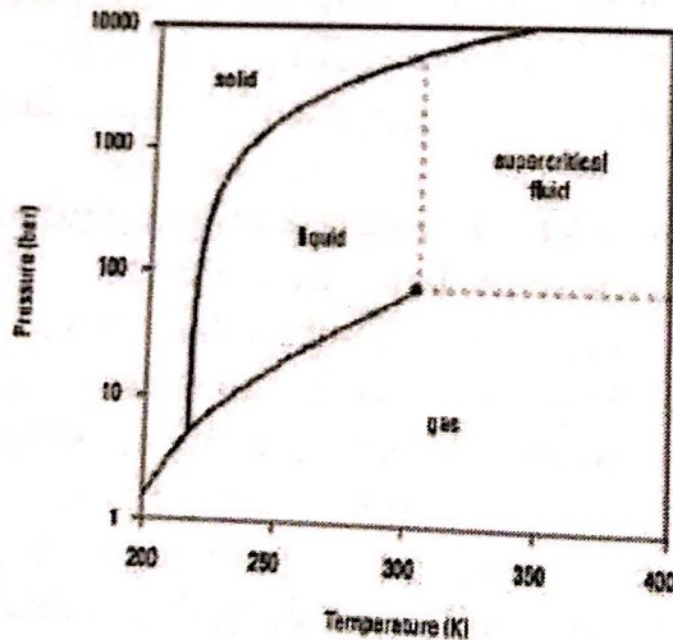
Gambar 13. Diagram hubungan temperatur-tekanan dari CO 2 sehingga dihasilkan cairan superkritis CO 2
