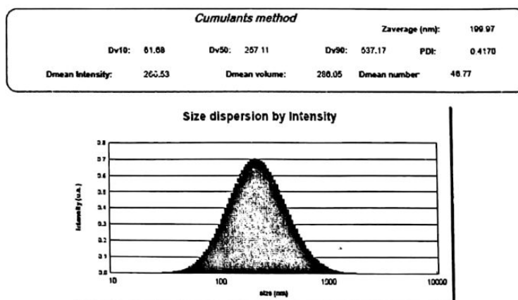
Gambar 2. Hasil pengukuran Particle Size Analyzer (PSA) 0,75 : 1 (g) (Fosfatidilkolin : Ekstrak Kulit Buah Kakao)
