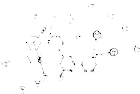
Gambar 4. Interaksi senyawa 13 terhadap protein 2IGX
