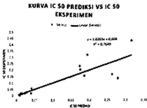
Gambar 2. Kurva hubungan aktivitas IC 50 eksperimen dan aktivitas IC 50 prediksi model persamaan terbaik
