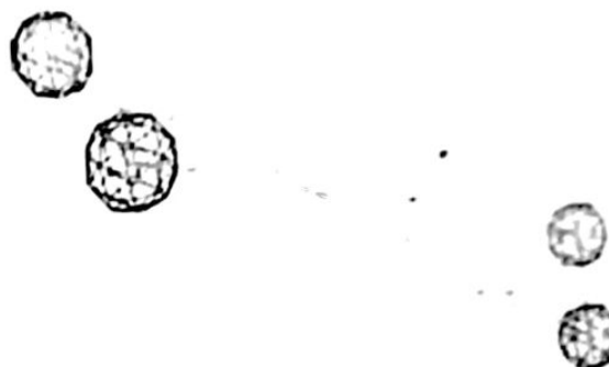
Gambar 6. jarak fitur farmakofor dalam query farmakofor
