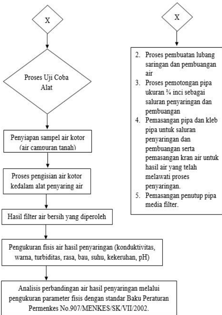
Gambar VIII.2: Flowchart perancangan dan pengujian alat
