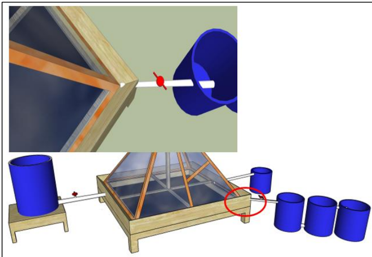
Gambar IV.4: Desain tempat keluarnya air hasil evaporasi ke wadah penampungan air evaporasi
