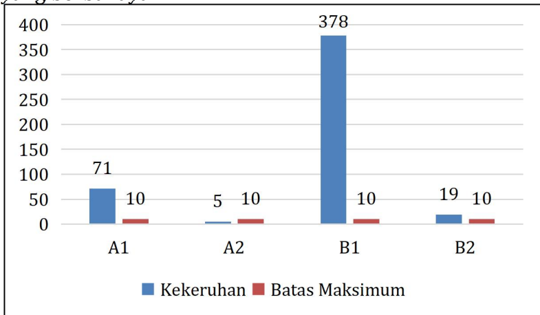
Gambar VIII.9: Grafik pengukuran kekeruhan/NTU sampel A dan B sebelum dan setelah penyaringan
