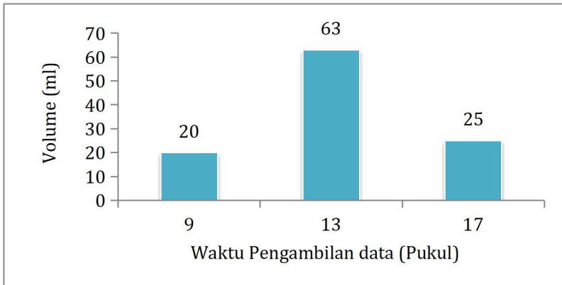
Gambar VI.13: Grafik volume air hasil destilasi rata-rata pada kemiringan wadah destilasi 4 0
