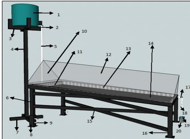
Gambar VI.1: Desain rancangan alat destilasi air laut
