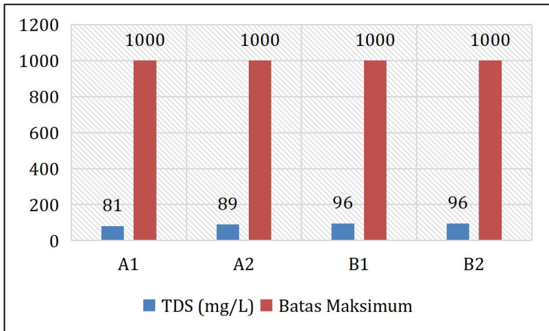
Gambar VIII.7: Grafik pengukuran jumlah zat terlarut/TDS sampel A dan B sebelum dan setelah penyaringan
