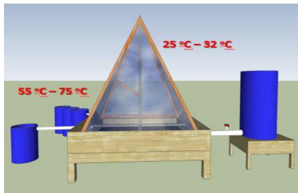
Gambar V.4: Kondisi suhu di dalam dan di luar piramida air
