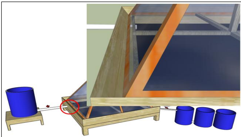
Gambar IV.2: Desain tempat masuknya aliran air baku ke dalam wadah penampungan alat
