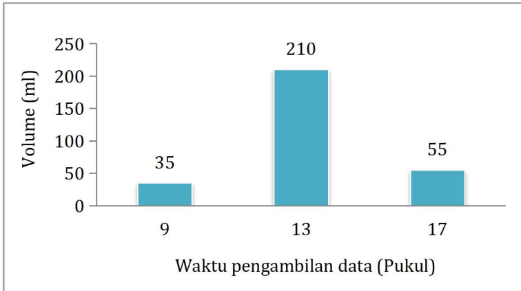
Gambar VI.12: Grafik volume air hasil evaporasi rata-rata pada kemiringan wadah destilasi 2 0
