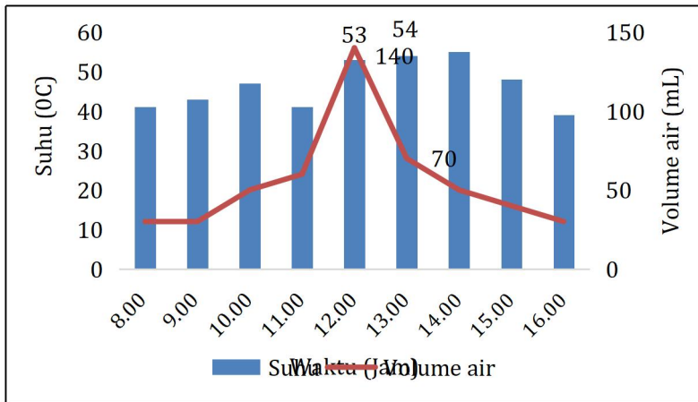
Gambar VII.11: Gambaran suhu dan volume air yang dihasilkan pada setiap waktu (08.00-16.00 wita) untuk Solar Still tipe piramida menggunakan kipas
