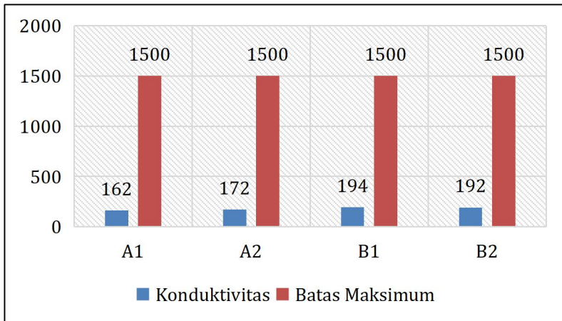
Gambar VIII.6: Grafik pengukuran konduktivitas sampel A dan B sebelum dan setelah penyaringan
