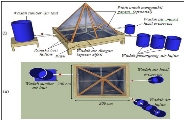
Gambar IV.1: Desain alat sistem pemurnian air laut menjadi air konsumsi menggunakan tenaga matahari (i) Tampak dari samping, (ii) Tampak dari atas
