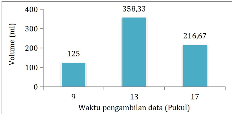
Gambar VI.15: Grafik volume air hasil destilasi rata-rata pada kemiringan wadah destilasi 2 0 dengan pengurangan debit aliran air dari penampungan
