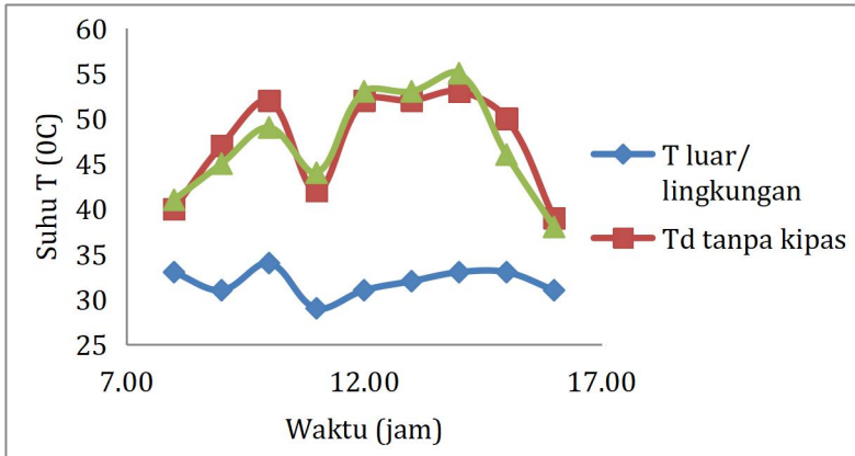
Gambar VII.10: Grafik distribusi temperatur Solar Still tipe prisma menggunakan kipas
