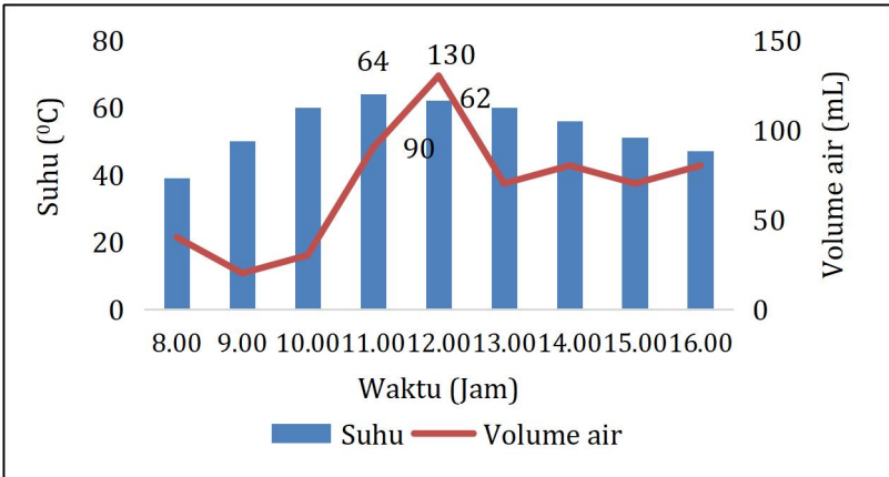
Gambar VII.7: Gambaran suhu dan volume air yang dihasilkan pada setiap waktu (08.00-16.00 wita) untuk solar still tipe piramida
