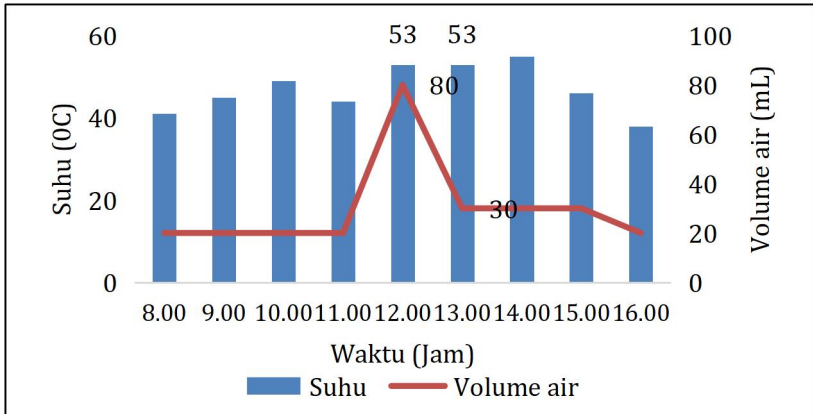
Gambar VII.12: Gambaran suhu dan volume air yang dihasilkan pada setiap waktu (08.00-16.00 wita) untuk Solar Still tipe prisma menggunakan kipas
