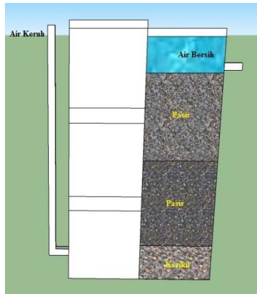
Gambar III.7: Saringan pasir cepat
