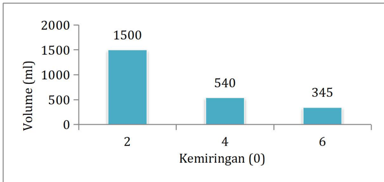
Gambar VI.16: Grafik Hubungan antara kemiringan dan volume air destilasi
