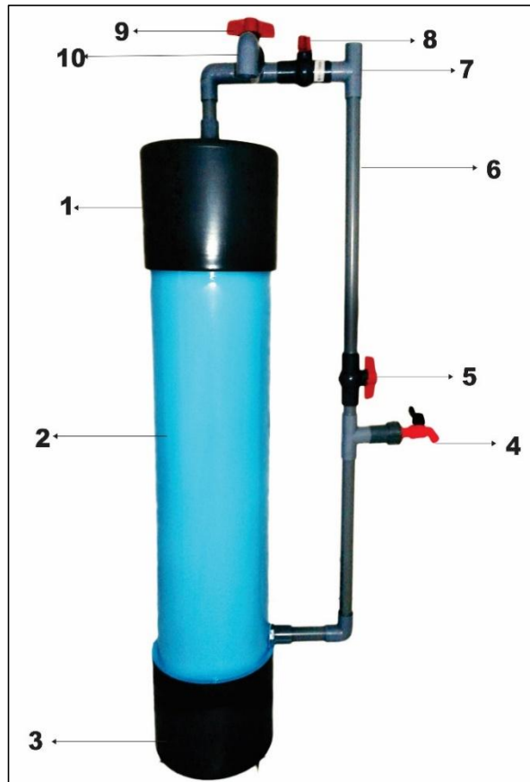
Gambar VIII.3: Hasil pembuatan alat penyaring air otomatis
