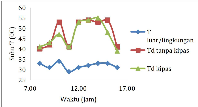
Gambar VII.9: Grafik distribusi temperatur Solar Still tipe piramida menggunakan kipas
