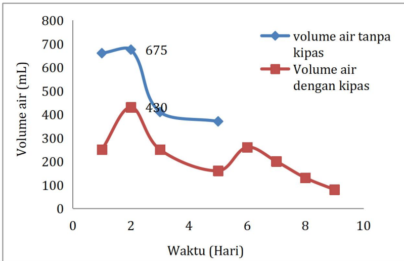
Grafik VII.14: Perbandingan Volume air yang dihasilkan Solar Still tipe prisma tanpa kipas (konvensional) dengan menggunakan kipas (modifikasi)
