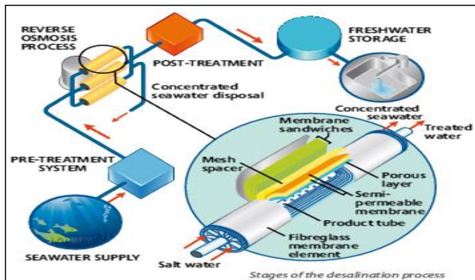
Gambar III.10: Skematik proses desalination dan reverse osmosis
