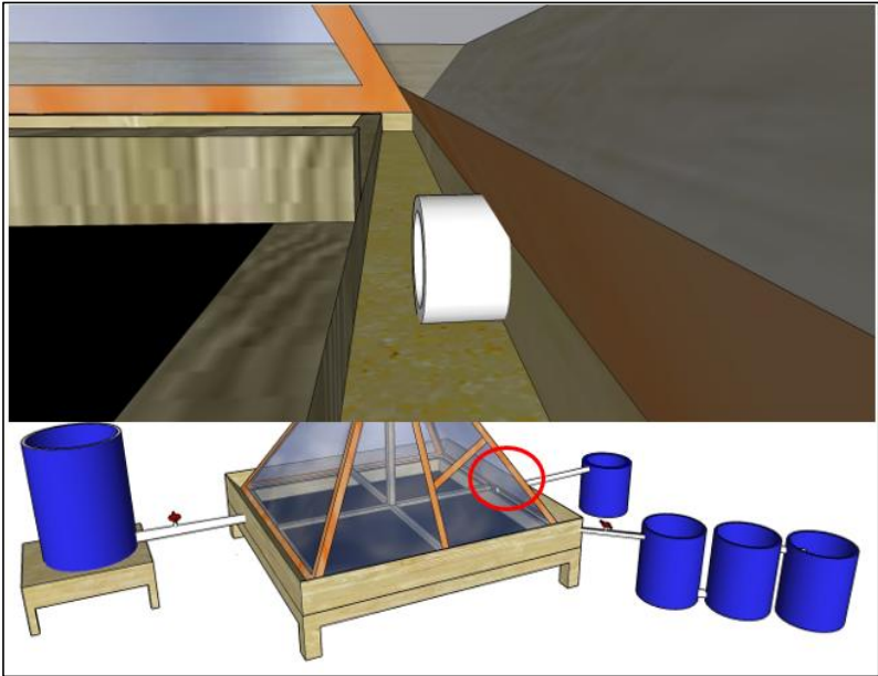
Gambar IV.3: Desain tempat aliran penampungan air hujan
