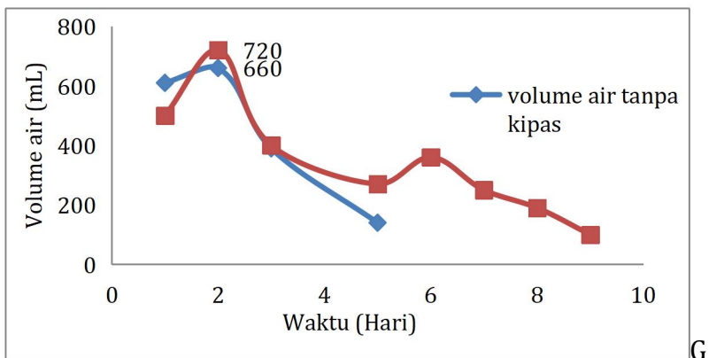
Gambar VII.13: Perbandingan volume air yang dihasilkan
