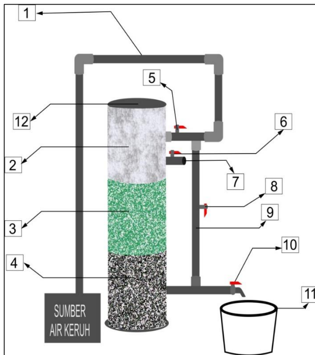
Gambar VIII.1: Rancang bangun alat penyaring air otomatis
