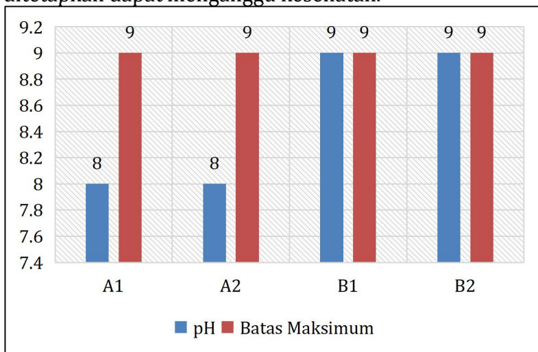
Gambar VIII.10: Grafik pengukuran pH ( Potensial of Hidrogen ) Sampel A dan B sebelum dan setelah penyaringan
