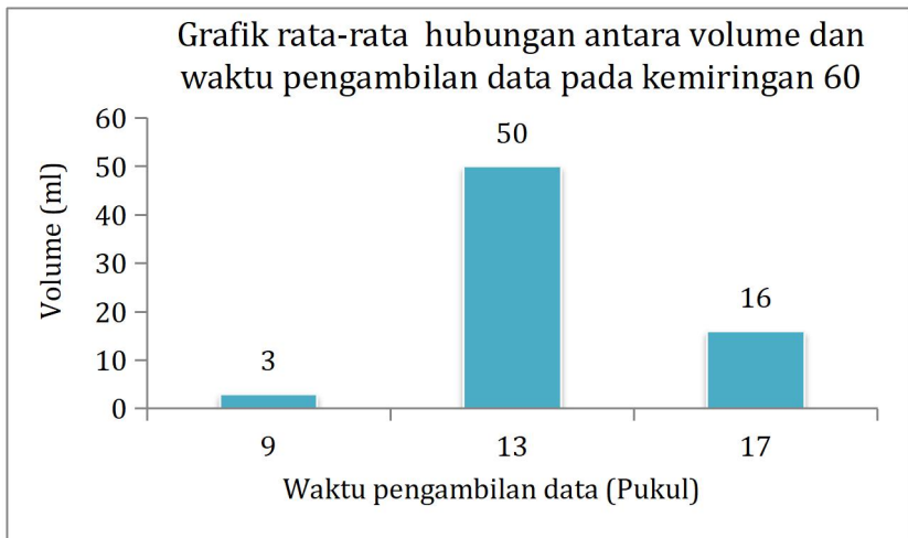
Gambar VI.12: Grafik volume air hasil destilasi rata-rata pada kemiringan wadah destilasi 6 0
