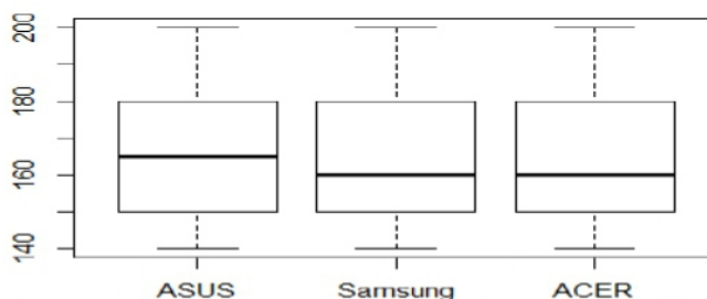
Gambar 9.1 Boxplot Permintaan Laptop
