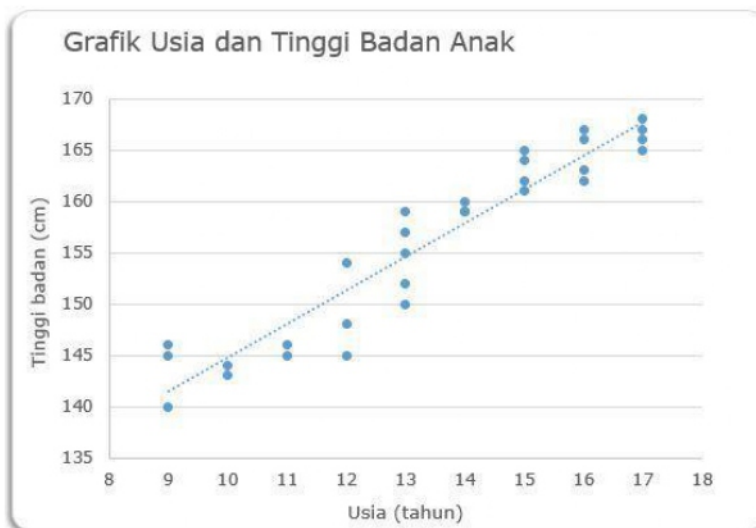
Gambar 7.1 Contoh Korelasi Positif
