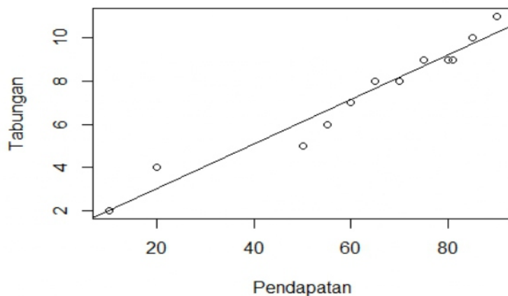
Gambar 7.3 Plot Pendapatan dan Tabungan
