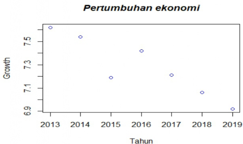
Gambar 4.8 Plot Type "p" Pertumbuhan ekonomi
