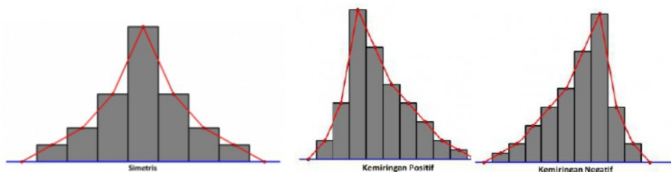
Gambar 5.1 Macam Model Ukuran Kemiringan
