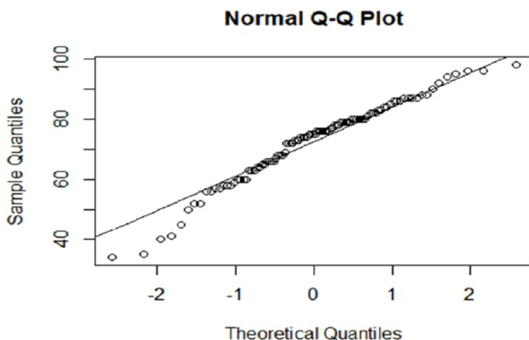
Gambar 6.2 Pengujian Normalitas Q – Q Plot
