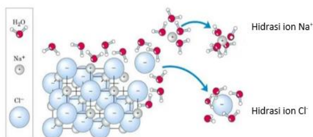
Gambar 7.1 Proses Hidrasi Ion \text{Na}^+ dan ion \text{Cl}^-
