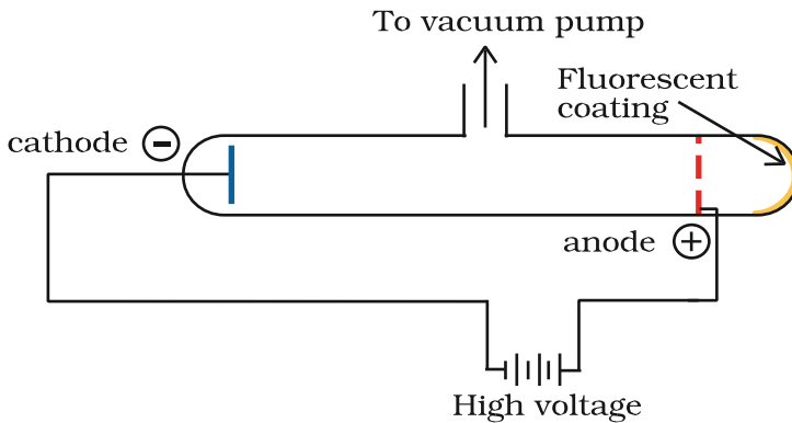
Gambar 2.1(b) Tabung pelepasan sinar katoda dengan anoda berlubang. Sumber: Anonim, Penaaksi.com
