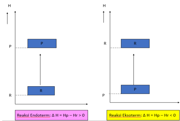
Gambar 8.2. Grafik Reaksi Eksoterm dan Endoterm (Evi, 2020)
