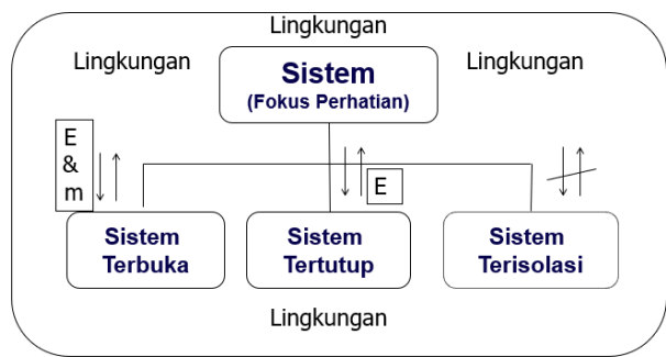
Gambar 8.1. Diagram Pertukaran Energi dan Materi Antara Sistem Terbuka, Sistem Tertutup, dan Sistem Terisolasi (Evi, 2020)
