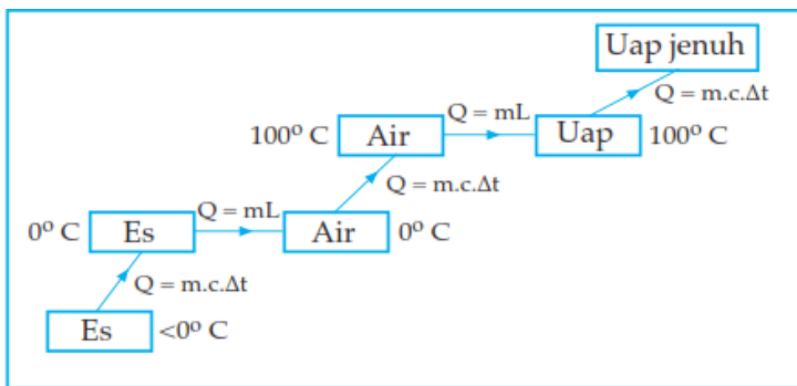
Gambar 6.6 Perubahan Wujud Zat Cair dan Kalor yang di Serap
