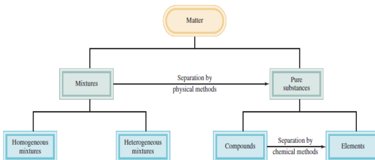
Gambar 6.1 Klasifikasi Materi (Raymond Chang, 2010)
