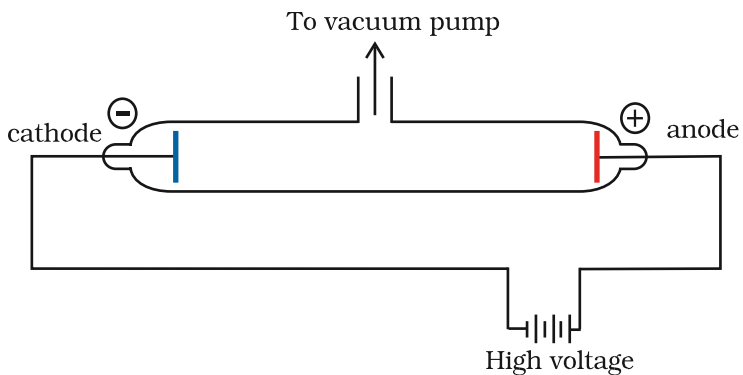
Gambar 2.1(a) Tabung pelepasan sinar katoda. Sumber: Anonim, Penaaksi.com
