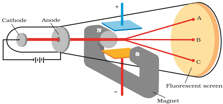
Gambar 2.2 Alat untuk menentukan rasio muatan terhadap massa electron. Sumber: Anonim, chem.co.id
