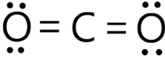
Gambar 5.3 Ikatan Kovalen Rangkap Dua
