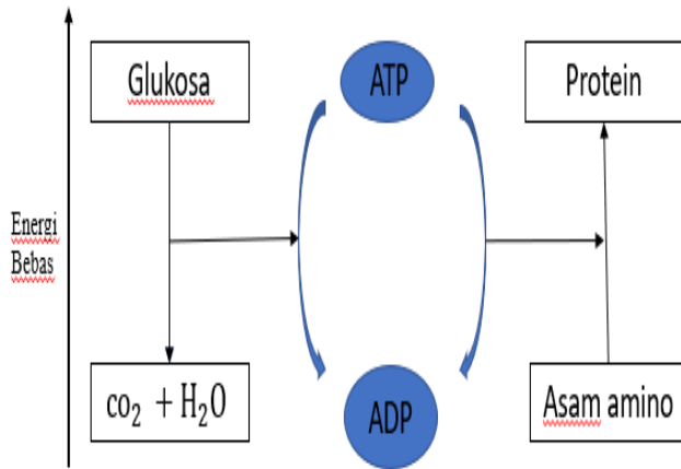
Gambar 8.3. Mekanisme Sintesis protein dari asam amino (Chang, 2004)
