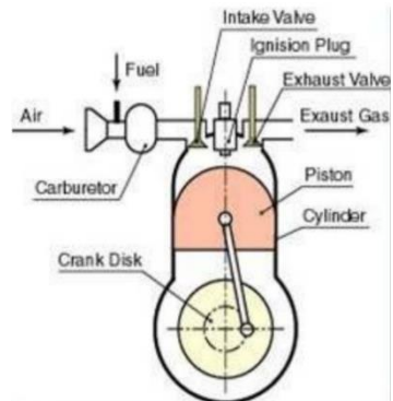
Gambar 8.6. Mesin kendaraan bermotor (Sumber: Analisa.id, 2020)
