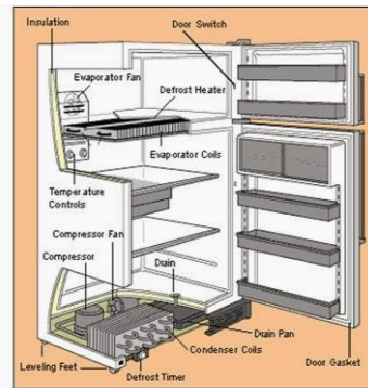
Gambar 8.5. Lemari es (Sumber: Mythermodynamicsblog, 2015)
