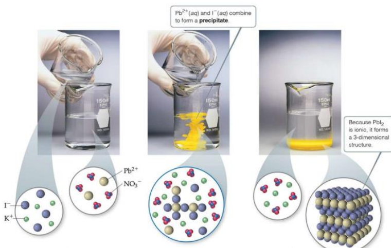
Gambar 3 Reaksi Pengendapan \text{PbI}_2
