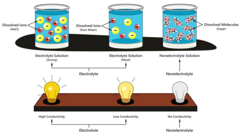
Gambar 7.2 Larutan Elektrolit (a) elektrolit kuat (b) elektrolit lemah (c) nonelektrolit
