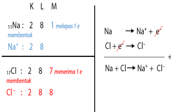
Gambar 1 contoh pembentukan senyawa ionic (Natrium Klorida) Sumber Anonim. https://idschool.net
