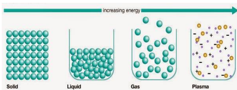
Gambar 6.3. Empat Wujud Zat (anonim/ https://www.britannica.com )
