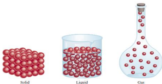
Gambar 6.2. Penampakan Mikroskopis Wujud Zat (Raymond Chang, 2010)
