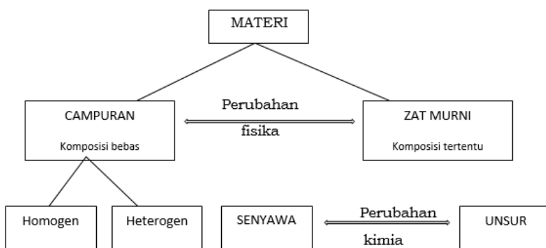
Gambar 1.1 Klasifikasi materi
