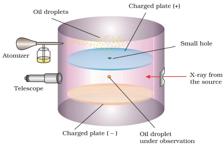
Gambar 2.3 Alat tetes minyak Millikan untuk mengukur muatan 'e'. Sumber: Anonim, chem.co.id
