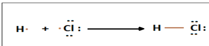
Gambar 5.2 Ikatan Kovalen Tunggal
