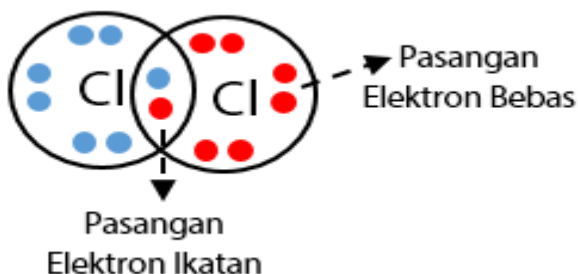
Gambar 5.1. Ikatan Kovalen Cl 2
