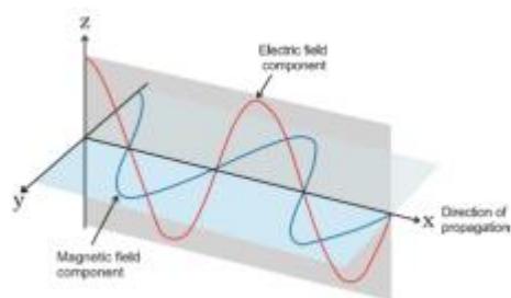
Gbr.2.6 Komponen medan listrik dan medan magnet gelombang elektromagnetik. Sumber: Anonim, chem.co.id
