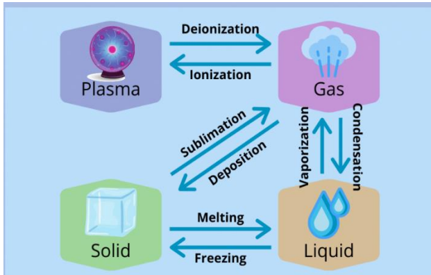
Gambar 6.5 Perubahan Wujud Zat (anonim/ https://sciencenotes.org )
