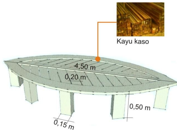
Gambar 4.21. Ukuran bangku taman dengan material kayu kaso (Sumber: Analisa penulis)
