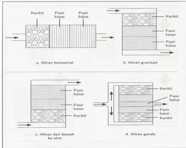
Gambar 2.11. Sistem penjernihan air dengan sistem filtrasi. (Sumber: Alamsjah, 2006)
