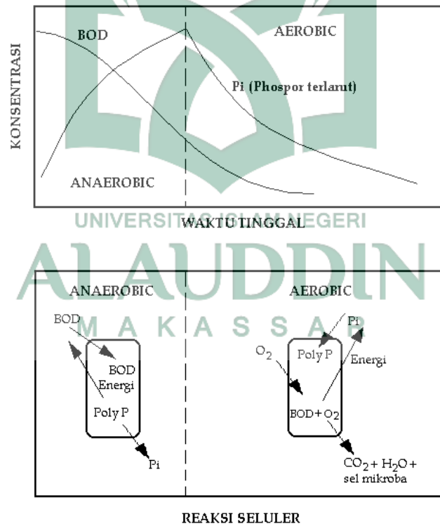
Gambar 2.9. Proses penghilangan fosfor oleh mikroorganisme di dalam proses pengolahan “Anaerob-Aerob”. (Sumber: Nusa Idaman Said, 2008)
