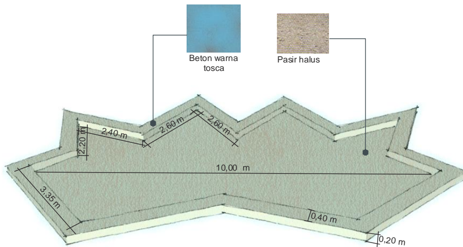
Gambar 4.8. Ukuran playground dengan material beton dan pasir halus (Sumber: Analisa penulis)
