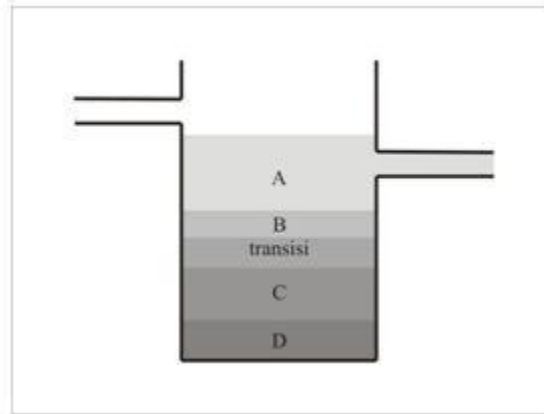
Gambar 2.20. Mekanisme sedimentasi kontinyu. (Sumber: Foust, 1980)
