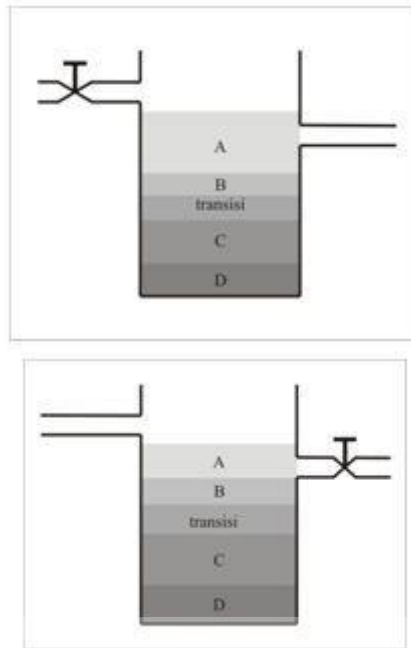
Gambar 2.19. Mekanisme sedimentasi semi-beach. (Sumber: Foust, 1980)
