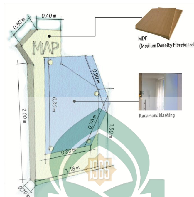
Gambar 4.16. Ukuran penanda peta dengan material MDF dan kaca sandblasting (Sumber: Analisa penulis)
