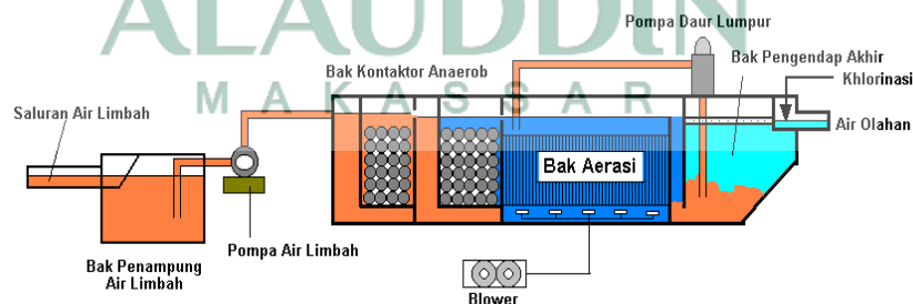
Gambar 2.5. Diagram proses pengolahan air limbah dengan proses aerasi kontak (Sumber: Nusa Idaman Said, 2008)
