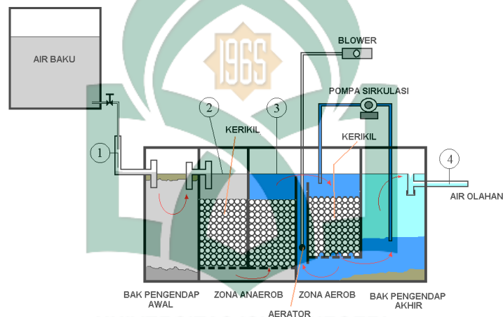
Gambar 2.8. Diagram proses pengolahan air limbah rumah tangga (domestik) dengan proses biofilter anaerob-aerob . (Sumber: Nusa Idaman Said, 2008)
