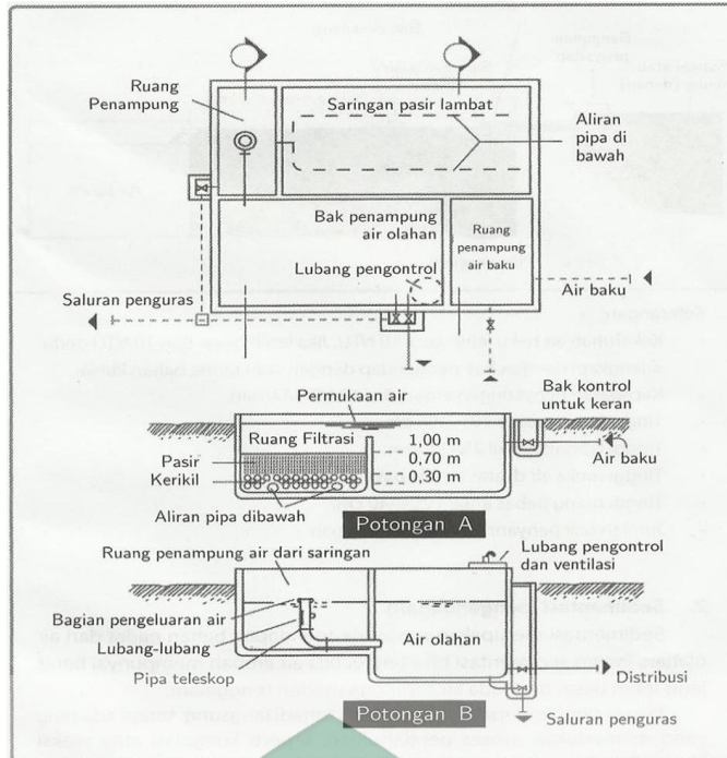
Gambar 2.14. Sistem penjernihan air dengan penyaringan pasir lambat. (Sumber: Alamsjah, 2006)
