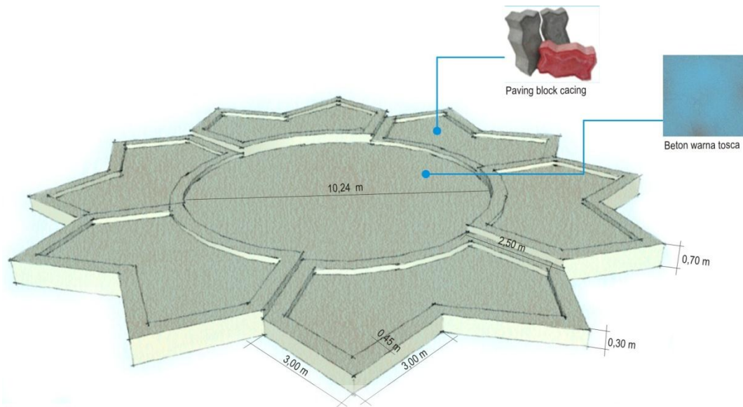
Gambar 4.10. Ukuran plaza dengan material paving block dan beton (Sumber: Analisa penulis)
