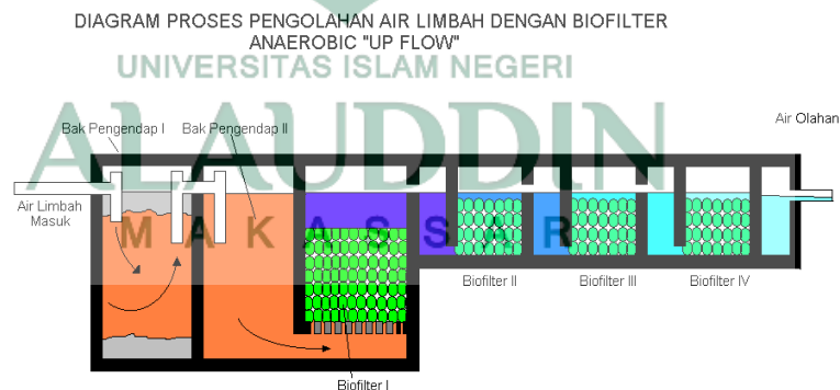
Gambar 2.6. Diagram proses pengolahan air limbah dengan sisten biofilter “Up flow”. (Sumber: Nusa Idaman Said, 2008)
