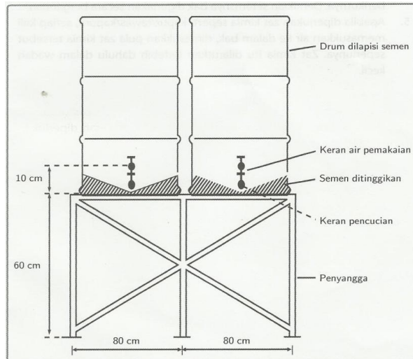
Gambar 2.16. Tempat sedimentasi air. (Sumber: Alamsjah, 2006)
