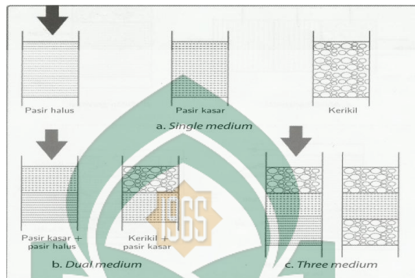
Gambar 2.10. sistem penjernihan air dengan saringan pasir. (Sumber: Alamsjah, 2006)
