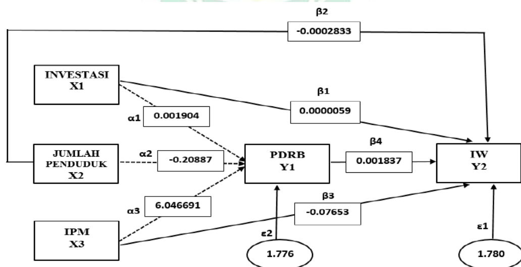
Gambar 4.2 Model Analisis Jalur
