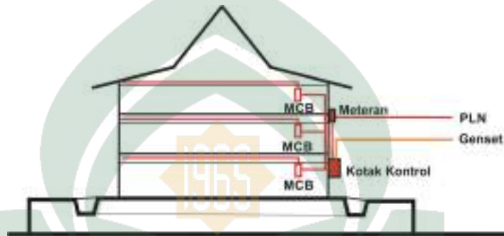
Gambar : Sistem Jaringan Listrik (Sumber. Olah Desain, 2020)
