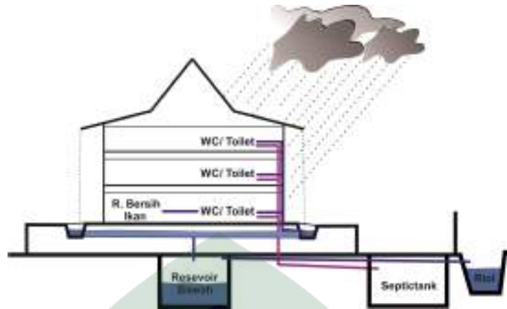
Gambar 34.1: Sistem Air Kotor (Sumber. Olah Desain, 2020)
