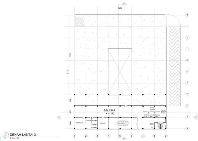
Gambar VI. 17 Denah Lantai 3 (Sumber: Hasil Desain, 2022)
