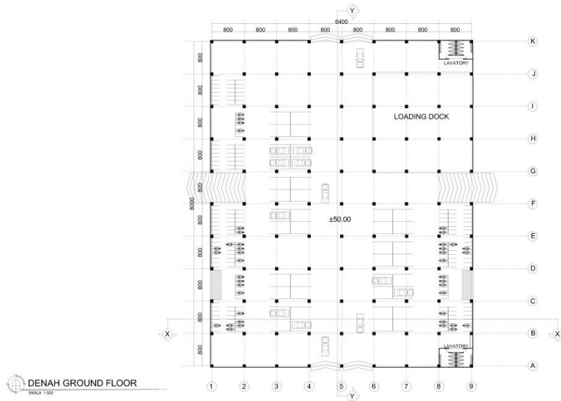
Gambar VI. 14 Denah Ground Floor (Sumber: Hasil Desain, 2022)
