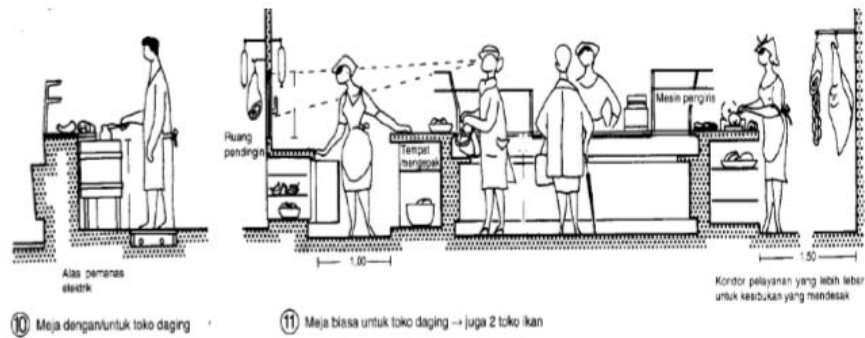
Gambar II. 4 Penataan Los Daging (Sumber: Data Arsitek Jilid 2, diakses 2020)
