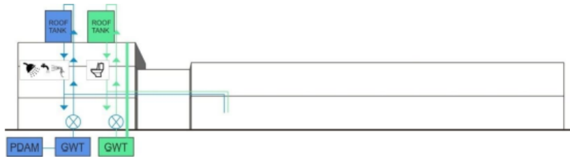
Gambar IV 3 Perencanaan Jaringan Air Bersih (Sumber: Olah Data, 2021)
