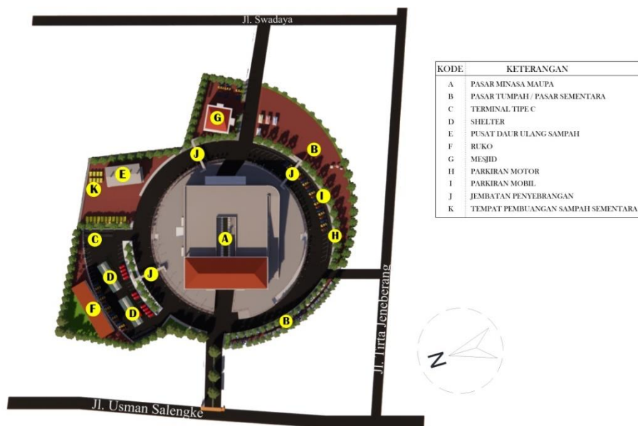
Gambar VI. 8 Masterplan (Sumber: Hasil Desain, 2022)
