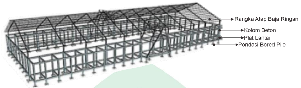
Gambar IV 2 Analisa Struktur (Sumber: Goggle, 2022)
