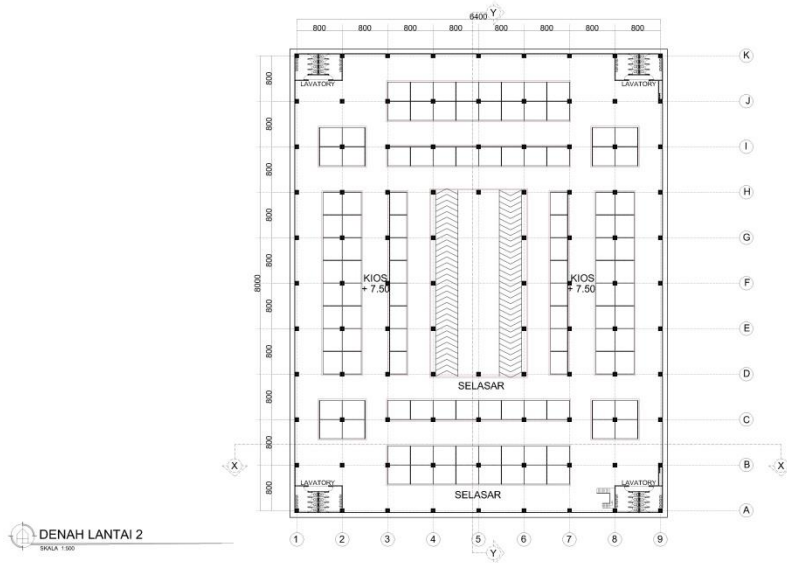
Gambar VI. 16 Denah Lantai 2 (Sumber: Hasil Desain, 2022)
