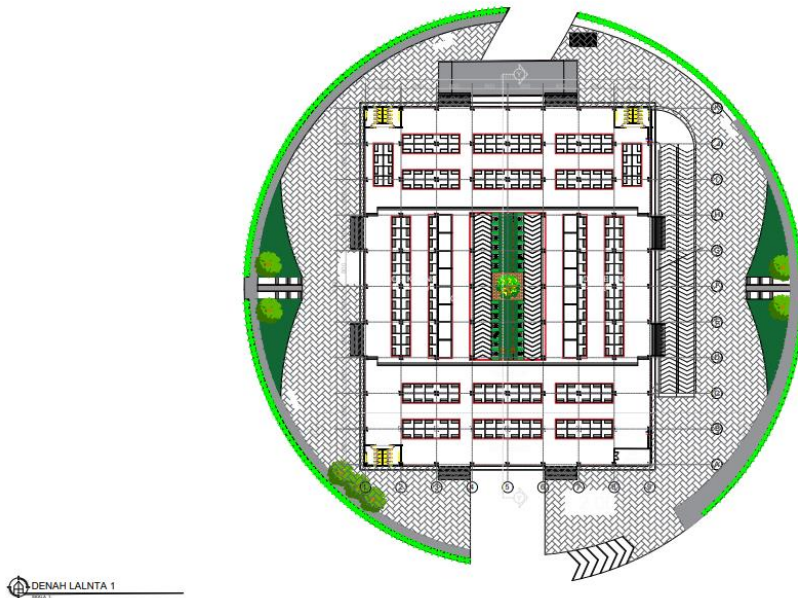
Gambar VI. 15 Denah Lantai 1 (Sumber: Hasil Desain, 2022)
