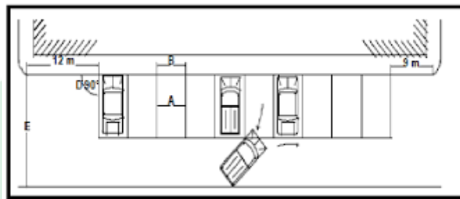
Gambar II. 8 Sistem Parkir Tegak Lurus
