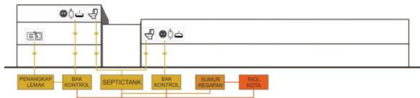
Gambar IV 4 Perencanaan Jaringan Air Kotor (Sumber: Olah Data, 2021)
