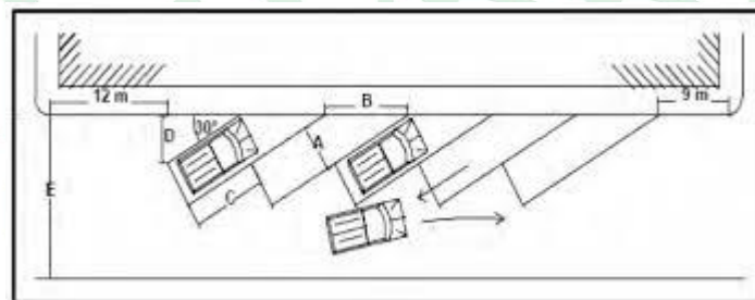
Gambar II. 9 Sistem Parkir Gergaji Lurus
