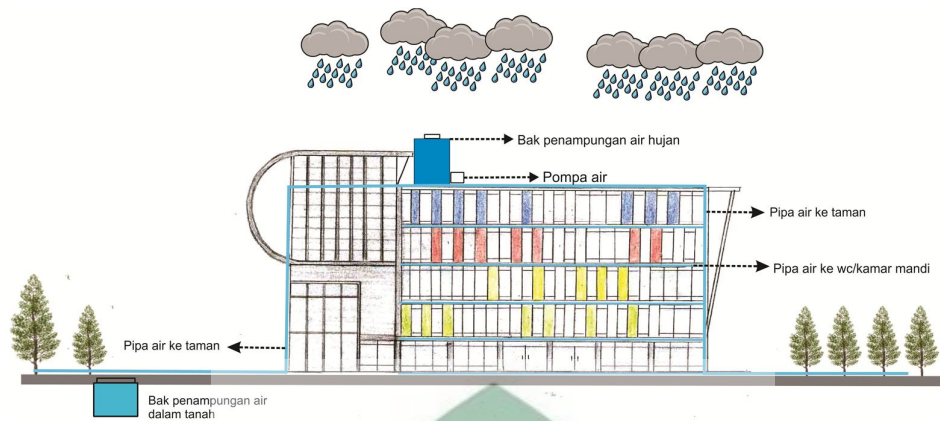
Gambar IV.32. Sistem air hujan (Dokumen Pribadi, 2014)
