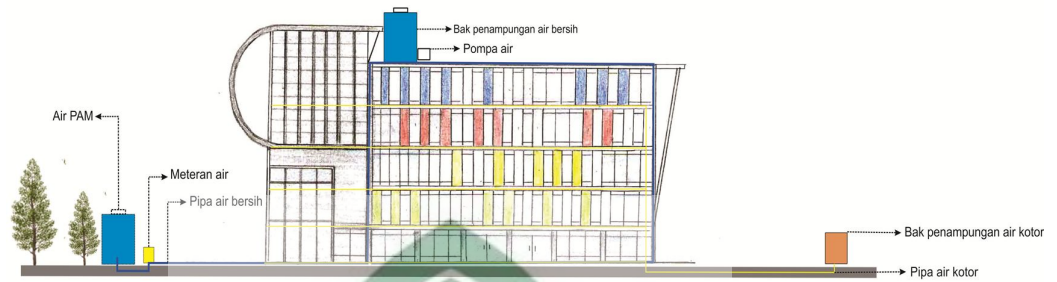
Gambar IV.30. Sistem air bersih (Dokumen Pribadi, 2014)
