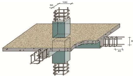
Gambar IV.22. Sistem balok dan kolom (Dokumen Pribadi, 2014)
