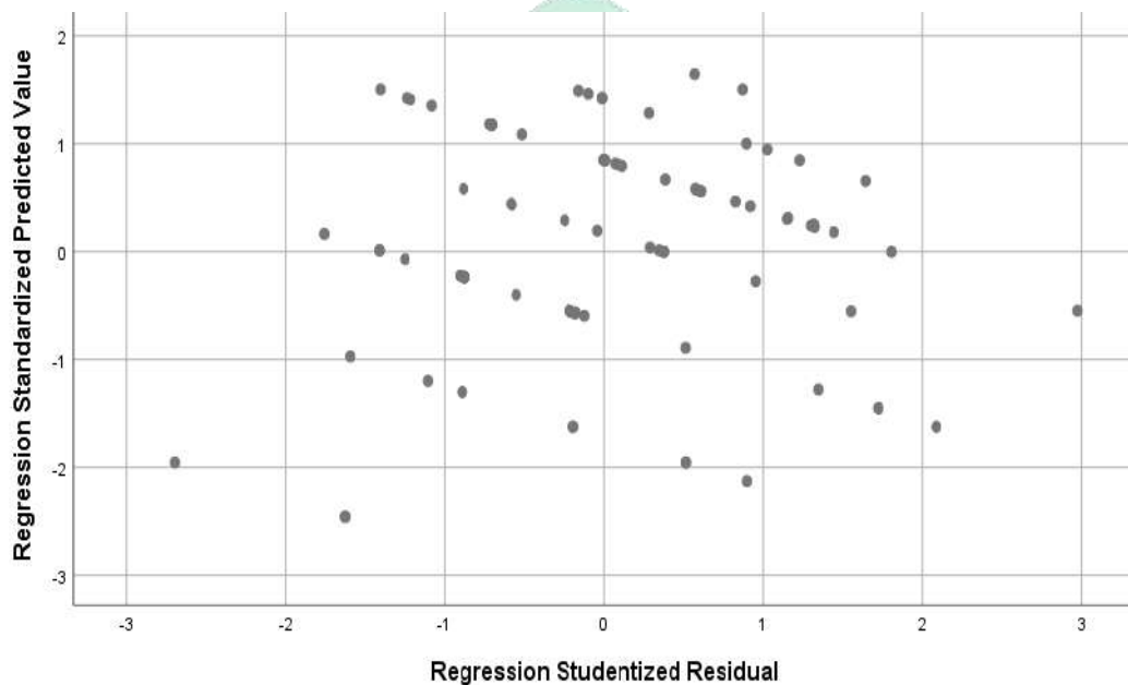
Gambar 4.1 Uji Heteroskedakitisitas
