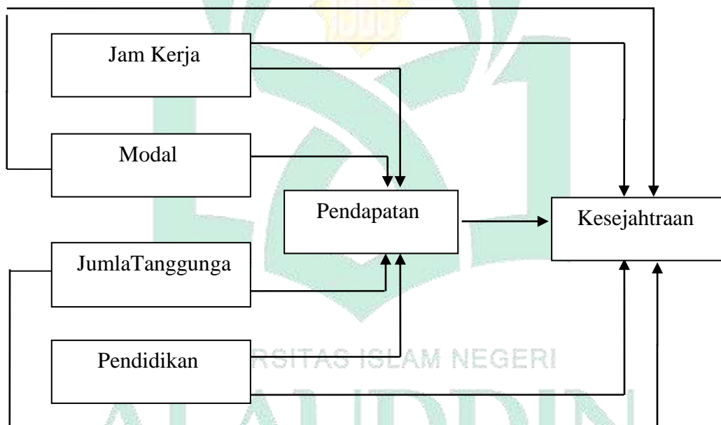
Gambar 2.1 Kerangka Pikir
