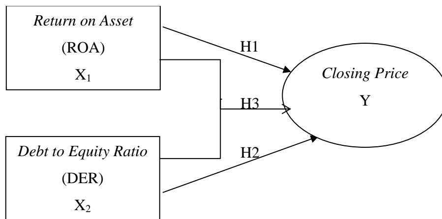
Gambar 2.1 Kerangka Pikir
