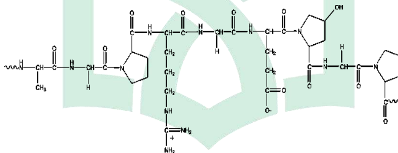
Gambar 2. Rumus struktur gelatin
