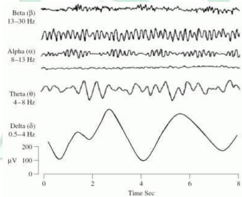
Gambar 2. Gelombang Otak
