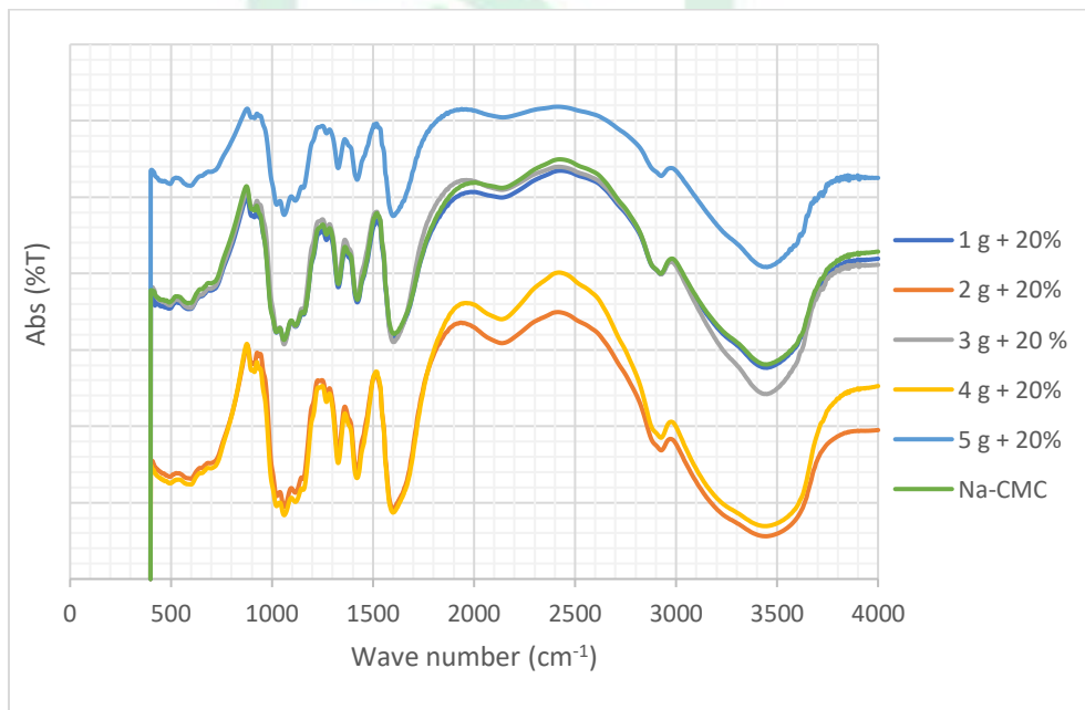
Gambar 13. Grafik Hasil Konsentrasi Variasi NaOH 20% dan Na MCA (1, 2, 3, 4, 5 g) menggunakan FTIR
