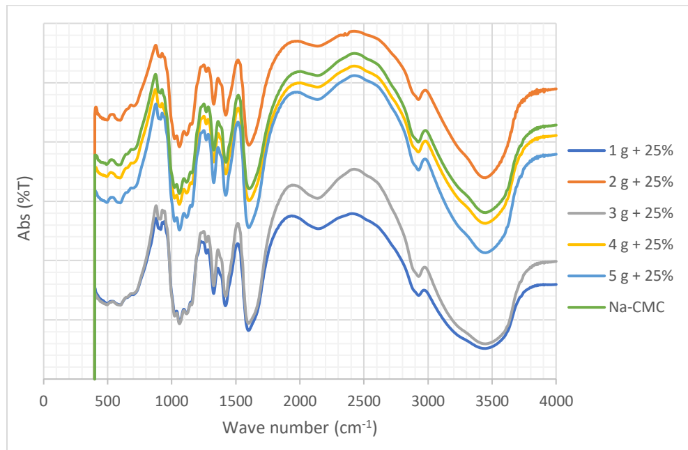
Gambar 14. Grafik Hasil Konsentrasi Variasi NaOH 25% dan Na MCA (1, 2, 3, 4, 5 g) menggunakan FTIR
