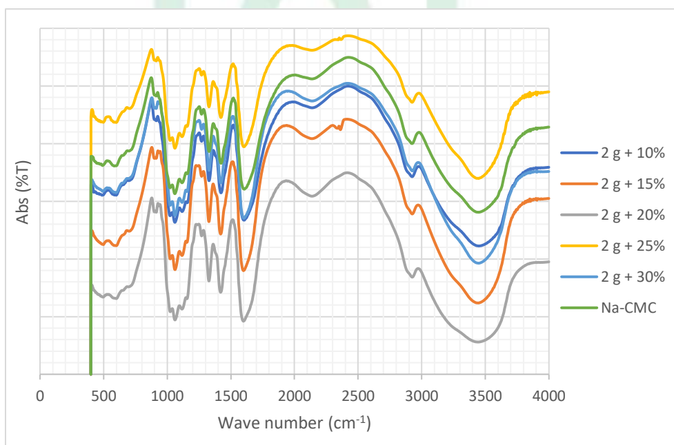
Gambar 7. Grafik Hasil Konsentrasi Variasi Na MCA 2 g dan NaOH(10, 15, 20, 25, 30%) menggunakan FTIR
