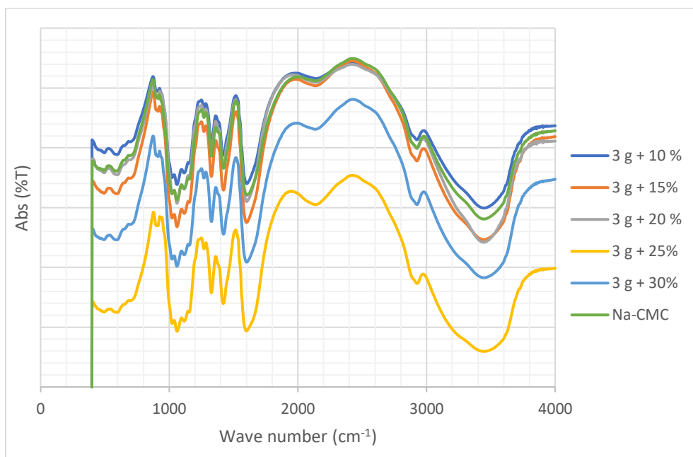
Gambar 8. Grafik Hasil Konsentrasi Variasi Na MCA 3 g dan NaOH (10, 15, 20, 25, 30%) menggunakan FTIR
