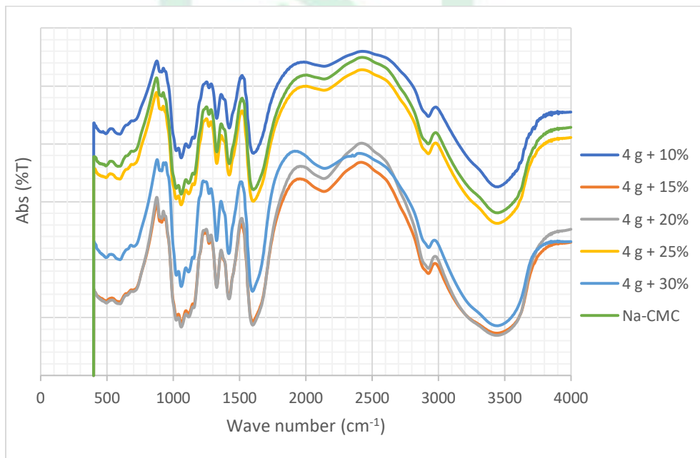
Gambar 9. Grafik Hasil Konsentrasi Variasi Na MCA 4 g dan NaOH (10, 15, 20, 25, 30%) menggunakan FTIR
