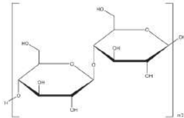
Gambar 3. Struktur Selulosa
