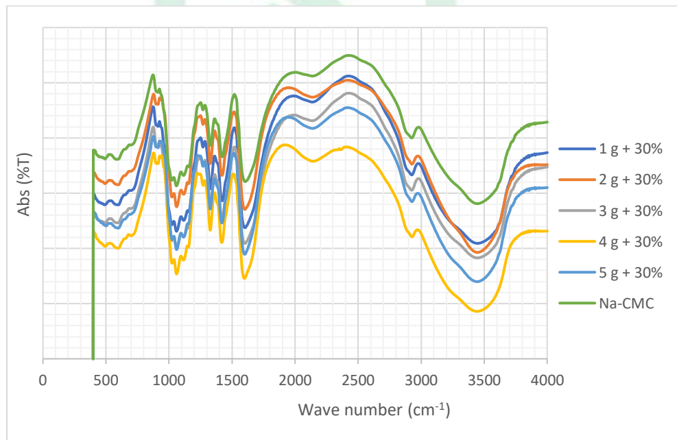
Gambar 15. Grafik Hasil Konsentrasi Variasi NaOH 30% dan Na MCA (1, 2, 3, 4, 5 g) menggunakan FTIR
