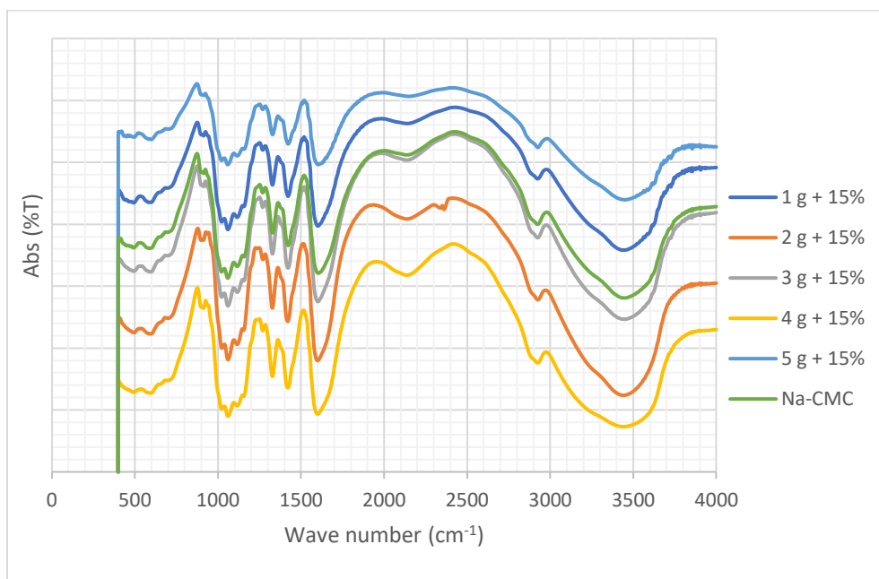
Gambar 12. Grafik Hasil Konsentrasi Variasi NaOH 15% dan Na MCA (1, 2, 3, 4, 5 g) menggunakan FTIR
