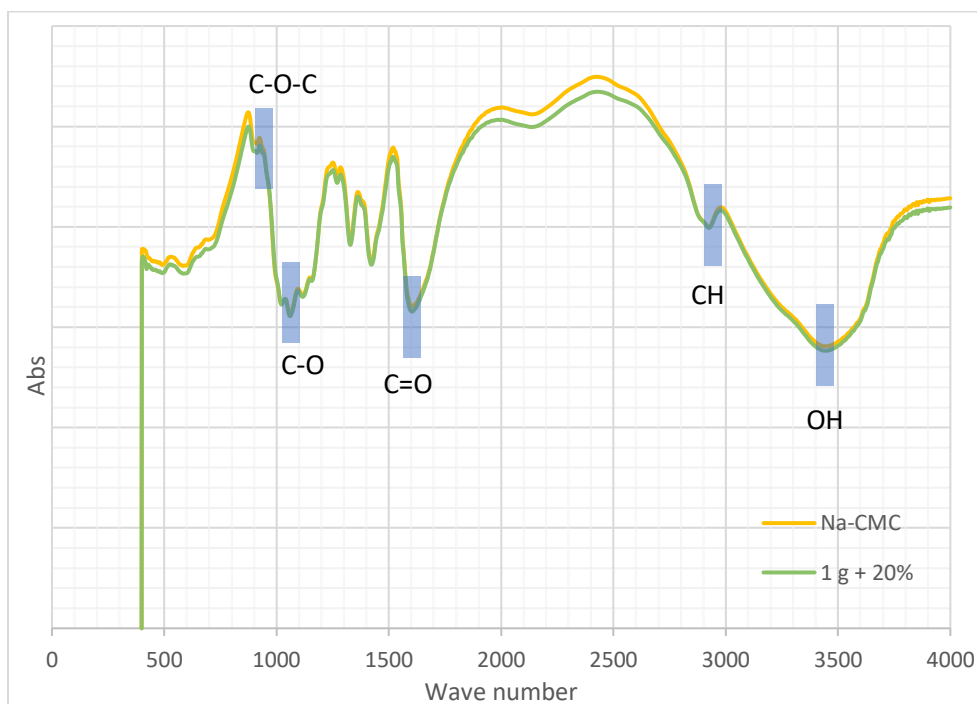
Gambar 16. Grafik Perbandingan Konsentrasi Variasi terbaik NaOH dan Na MCA menggunakan FTIR
