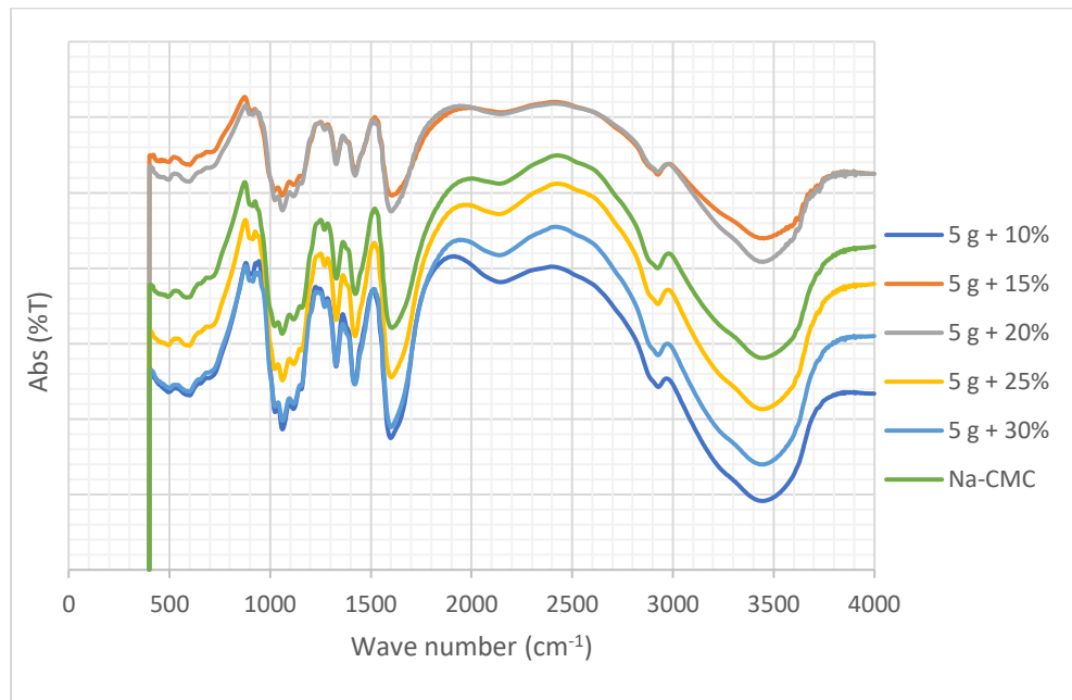
Gambar 10. Grafik Hasil Konsentrasi Variasi Na MCA 5 g dan NaOH (10, 15, 20, 25, 30%) menggunakan FTIR
