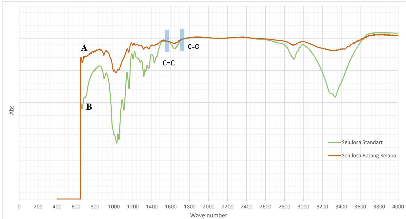
Gambar 5. Hasil analisis gugus fungsi selulosa menggunakan FTIR A) Selulosa Batang Kelapa, B) Selulosa Standart
