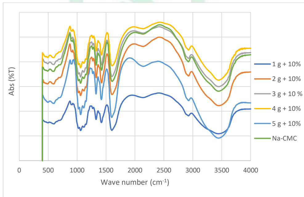
Gambar 11. Grafik Hasil Konsentrasi Variasi NaOH 10% dan Na MCA (1, 2, 3, 4, 5 g) menggunakan FTIR
