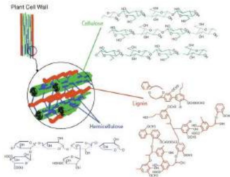
Gambar 2. Lignoselulosa
