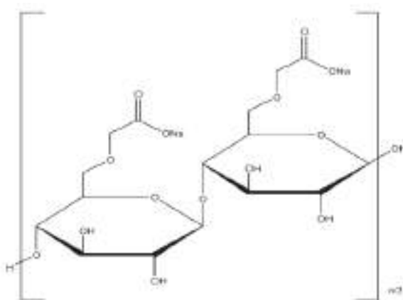
Gambar 4. Struktur Na-CMC
