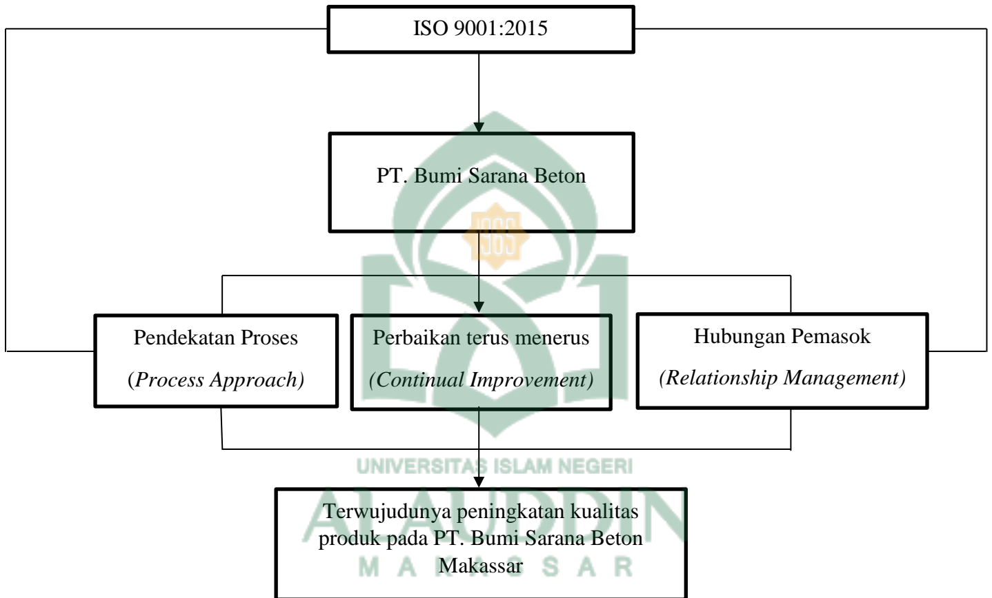
Gambar 2. 1 Kerangka Konseptual
