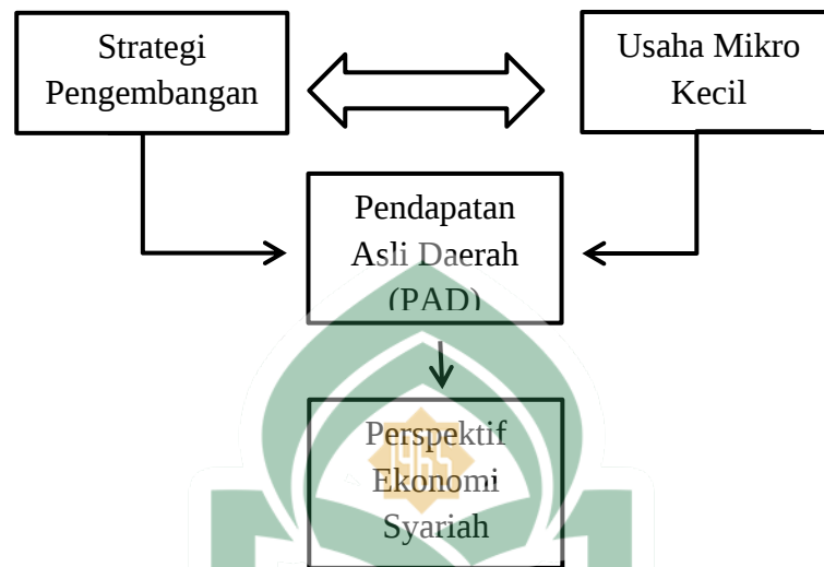
Gambar 2.1 Kerangka Konseptual
