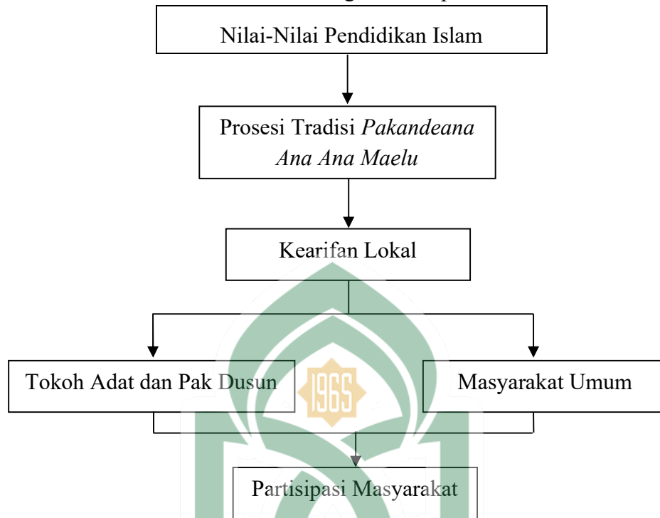
Gambar 1: Kerangka Konseptual
