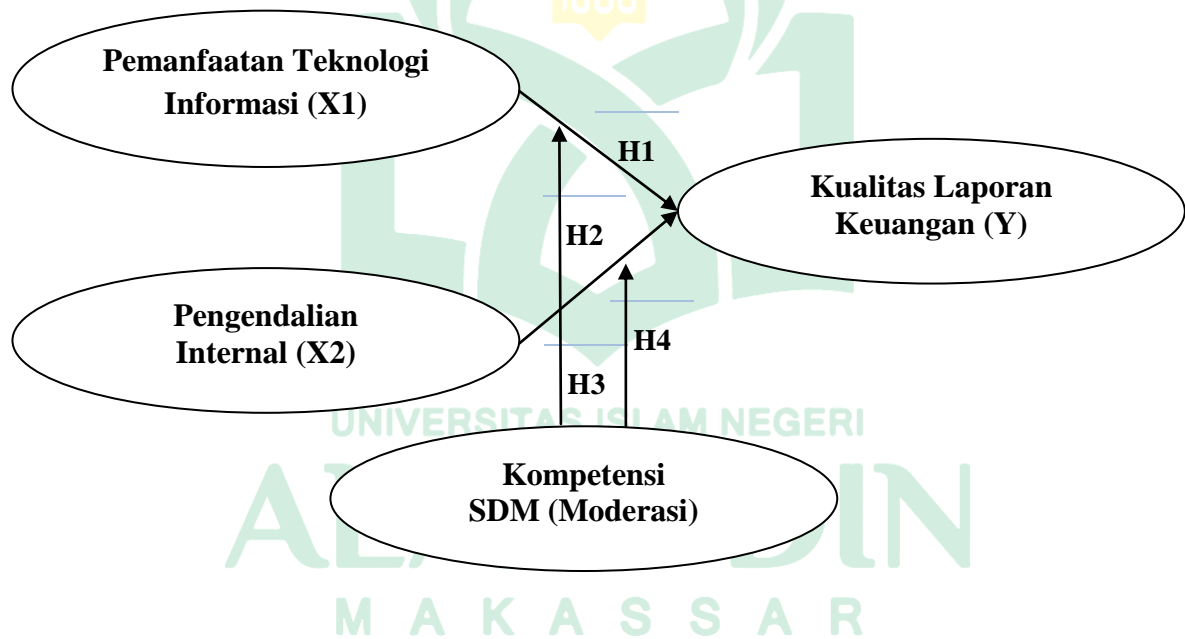
Gambar 2. 1 Kerangka Konseptual
