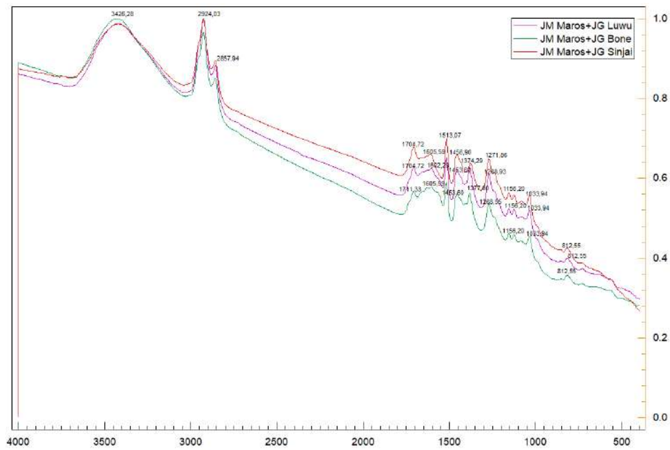
Gambar 4. 23. Spektrum Kombinasi Jahe Merah Maros dan Jahe Gajah Bone, Jahe Gajah Luwu, dan Jahe Gajah Sinjai
