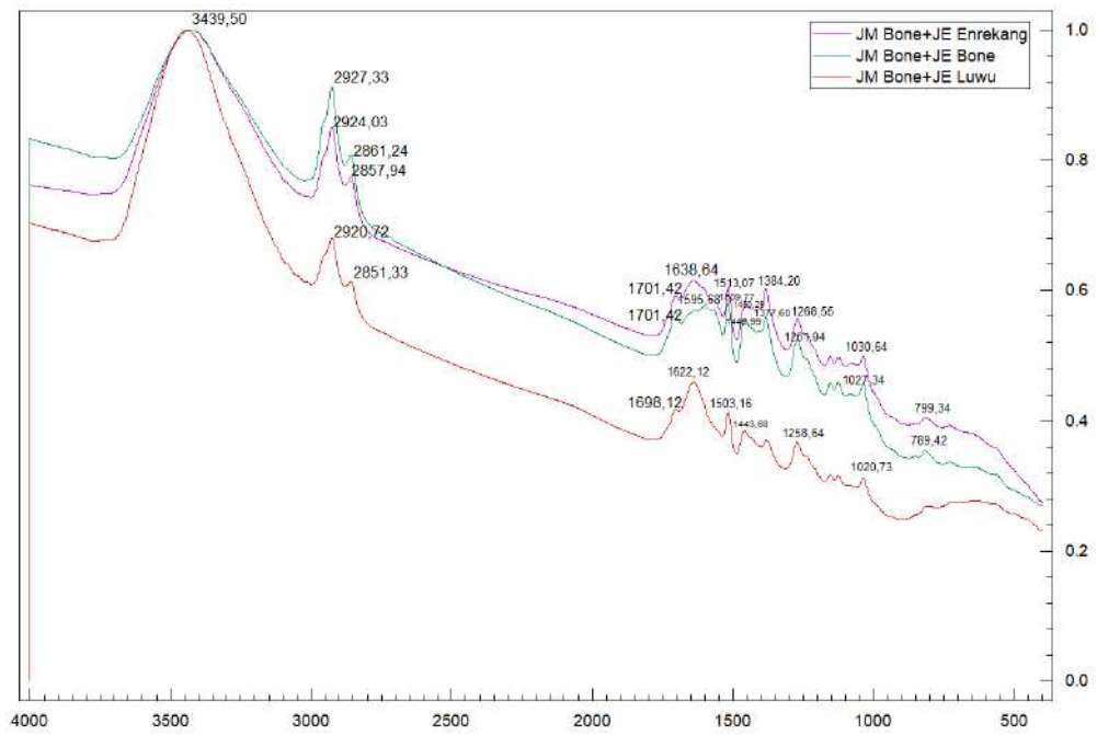
Gambar 4. 19. Spektrum Kombinasi Jahe Merah Bone dan Jahe Emprit Enrekang, Jahe Emprit Bone, dan Jahe Emprit Luwu
