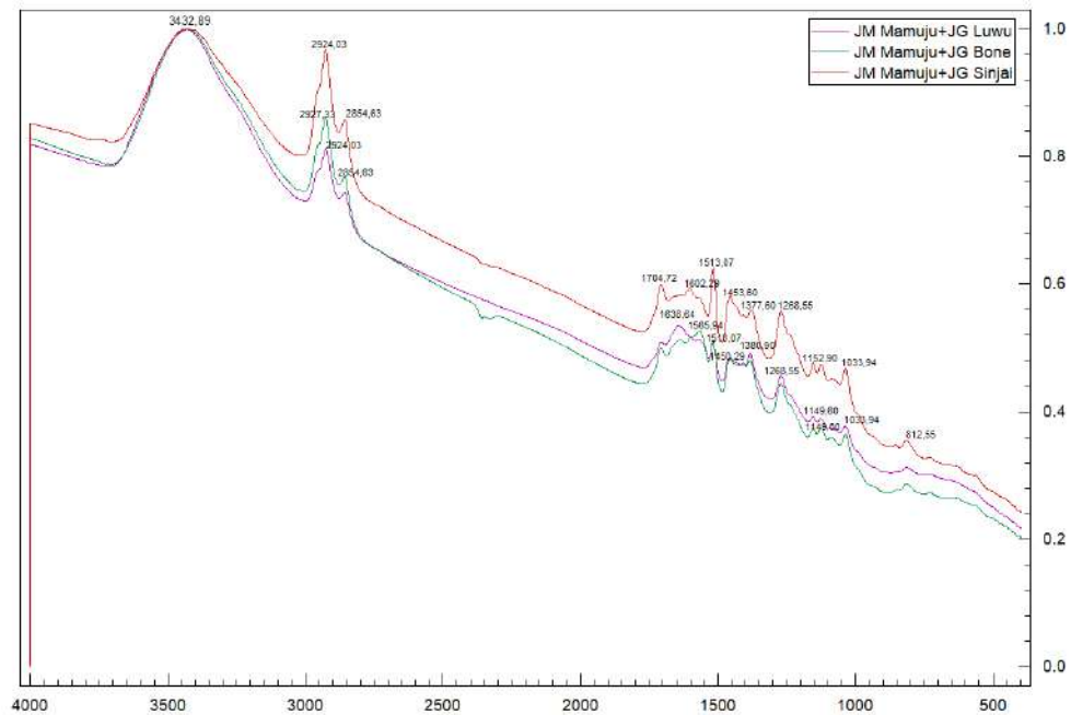
Gambar 4. 22. Spektrum Kombinasi Jahe Merah Mamuju dan Jahe Gajah Bone, Jahe Gajah Luwu, dan Jahe Gajah Sinjai
