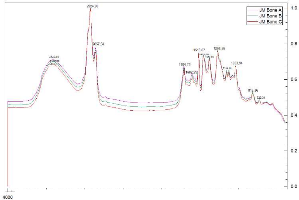
Gambar 4. 2. Spektrum Jahe Merah Bone
