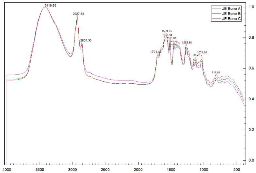
Gambar 4. 11. Spektrum Jahe Emprit Bone
