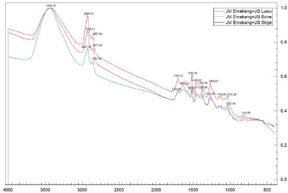
Gambar 4. 25. Spektrum Kombinasi Jahe Merah Enrekang dan Jahe Gajah Bone, Jahe Gajah Luwu, dan Jahe Gajah Sinjai
