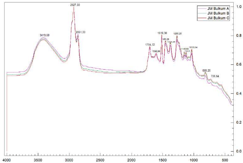
Gambar 4. 7 Spektrum Jahe Gajah Bone
