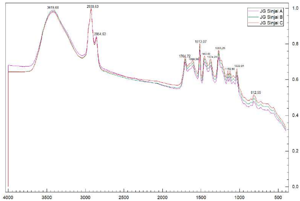
Gambar 4. 9. Spektrum Jahe Gajah Sinjai
