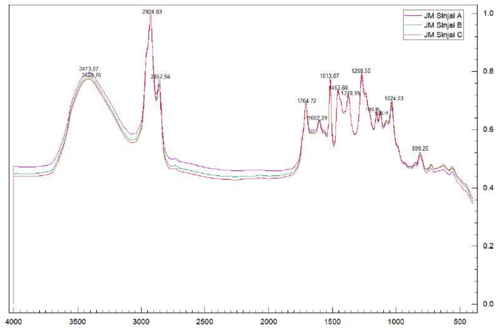
Gambar 4. 3 Spektrum Jahe Merah Sinjai
