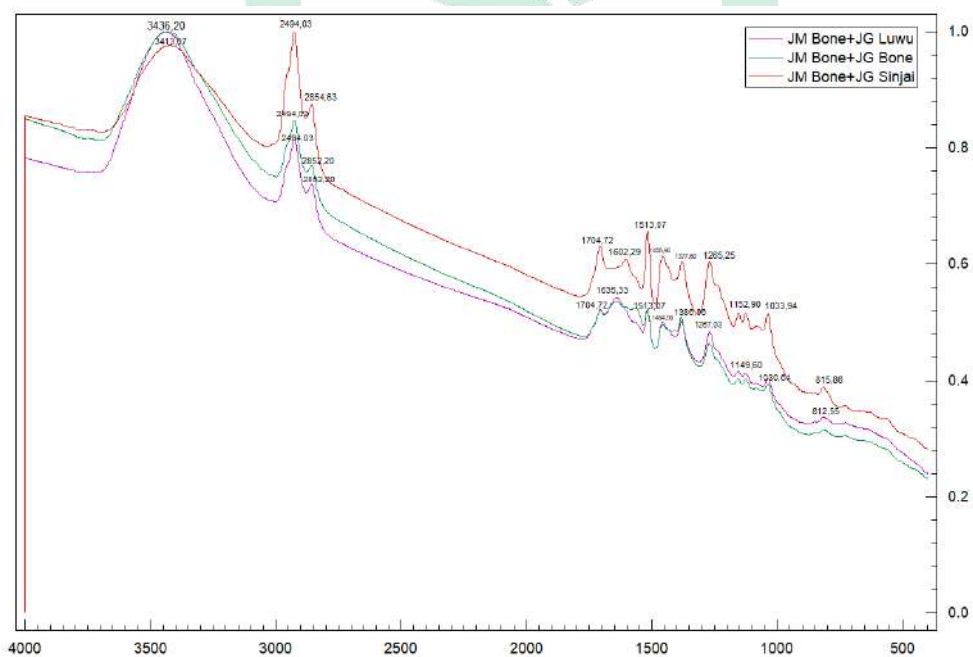
Gambar 4. 26. Spektrum Kombinasi Jahe Merah Bone dan Jahe Gajah Bone, Jahe Gajah Luwu, dan Jahe Gajah Sinjai
