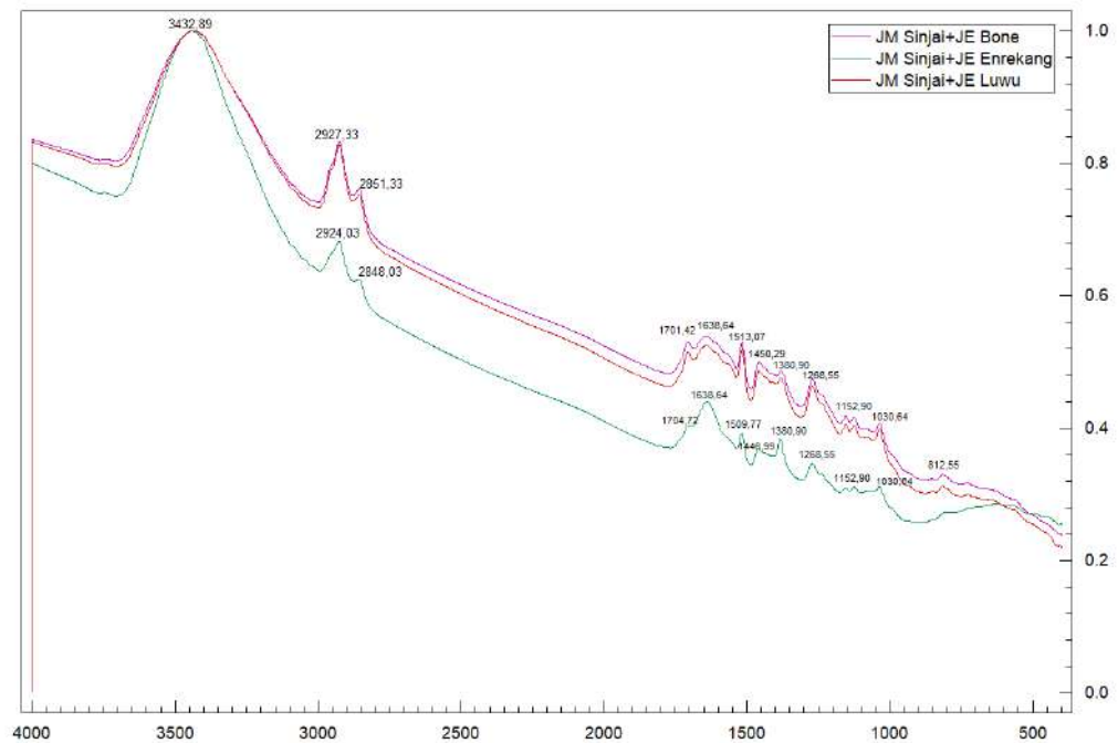
Gambar 4. 20. Spektrum Kombinasi Jahe Merah Sinjai dan Jahe Emprit Enrekang, Jahe Emprit Bone, dan Jahe Emprit Luwu.
