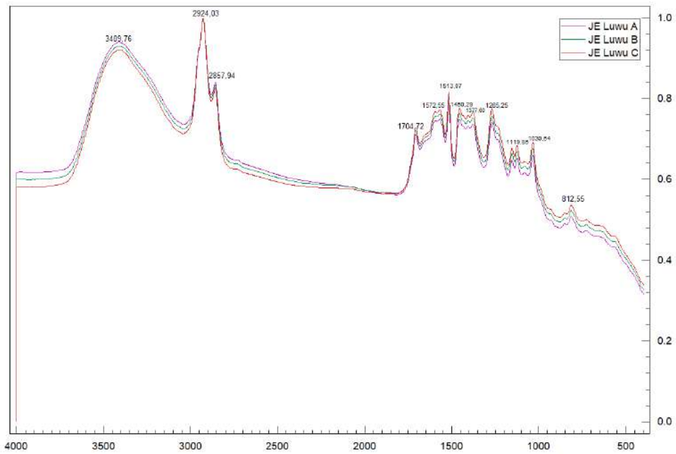
Gambar 4. 13. Spektrum Jahe Emprit Luwu
