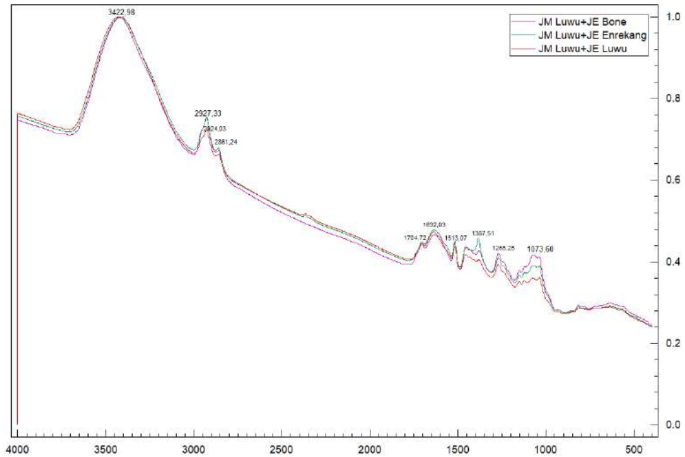
Gambar 4. 17. Spektrum Kombinasi Jahe Merah Luwu dan Jahe Emprit Enrekang, Jahe Emprit Bone, dan Jahe Emprit Luwu
