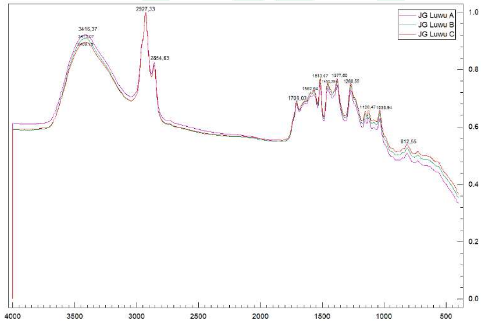
Gambar 4. 10. Spektrum Jahe Gajah Luwu
