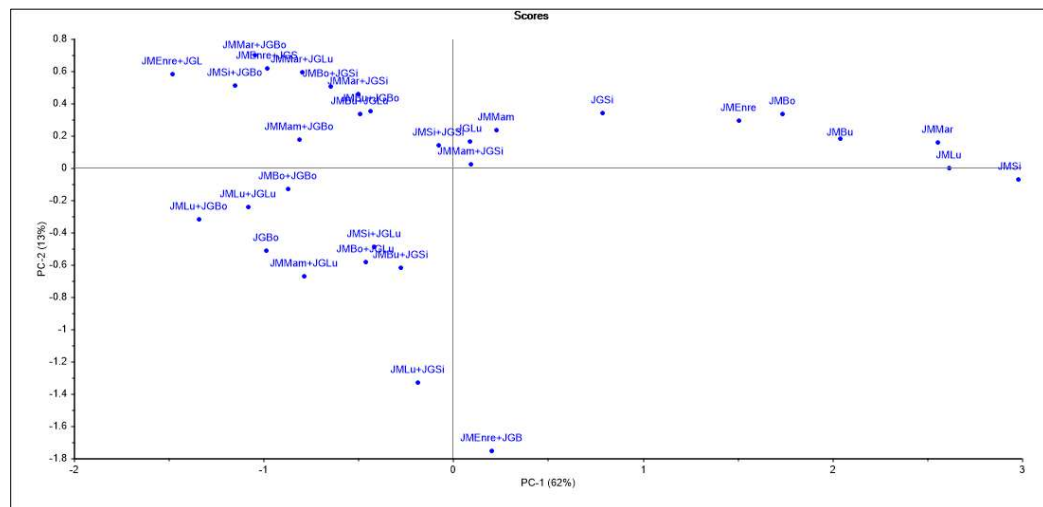
Gambar 4. 30. Score Plot PCA PC-1 dan PC-2 Jahe Merah dan Jahe Gajah Kombinasi
