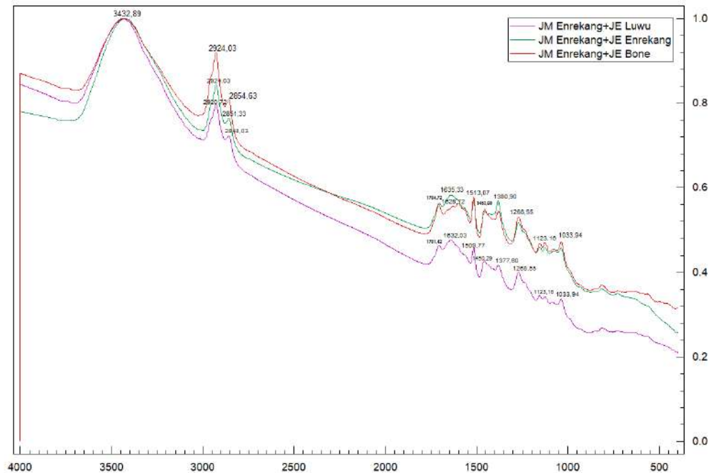
Gambar 4. 18. Spektrum Kombinasi Jahe Merah Enrekang dan Jahe Emprit Enrekang, Jahe Emprit Bone, dan Jahe Emprit Luwu
