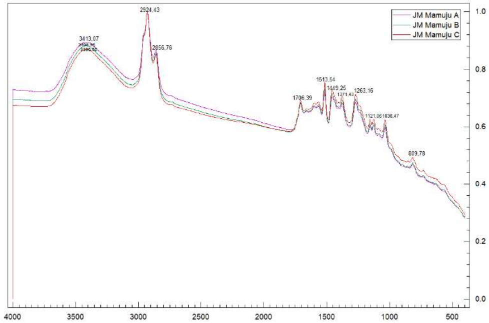
Gambar 4. 1. Spektrum Jahe Merah Mamuju
