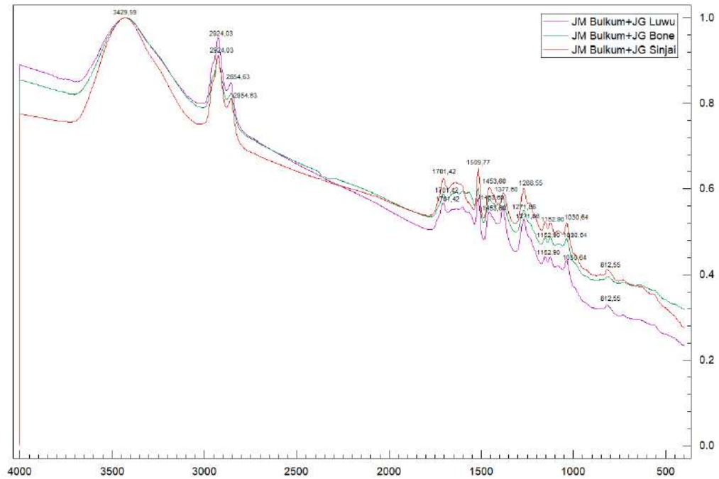
Gambar 4. 21. Spektrum Kombinasi Jahe Merah Bulukumba dan Jahe Gajah Bone, Jahe Gajah Luwu, dan Jahe Gajah Sinjai
