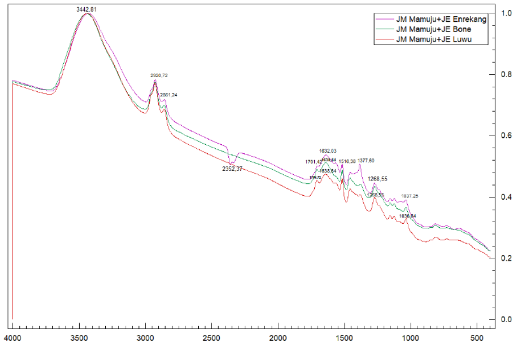
Gambar 4. 15. Spektrum Kombinasi Jahe Merah Mamuju dan Jahe Emprit Enrekang, Jahe Emprit Bone, dan Jahe Emprit Luwu
