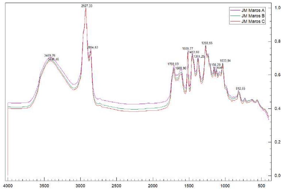
Gambar 4. 5. Spektrum Jahe Merah Maros
