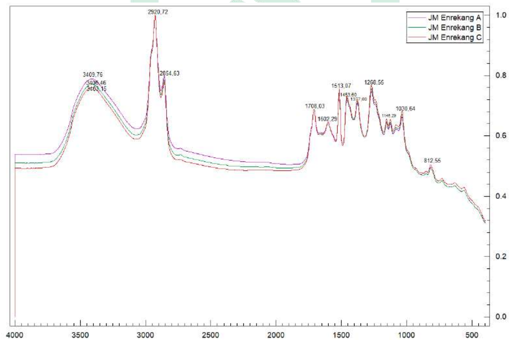
Gambar 4. 6. Spektrum Jahe Merah Enrekang
