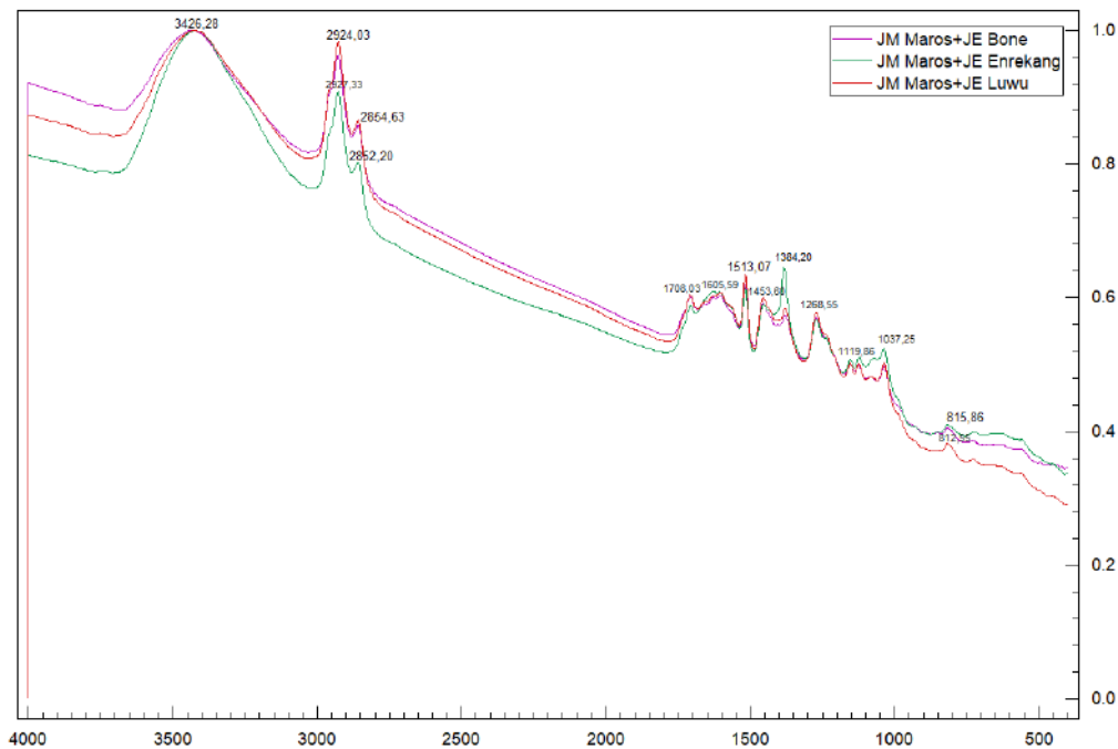
Gambar 4. 16. Spektrum Kombinasi Jahe Merah Maros dan Jahe Emprit Enrekang, Jahe Emprit Bone, dan Jahe Emprit Luwu
