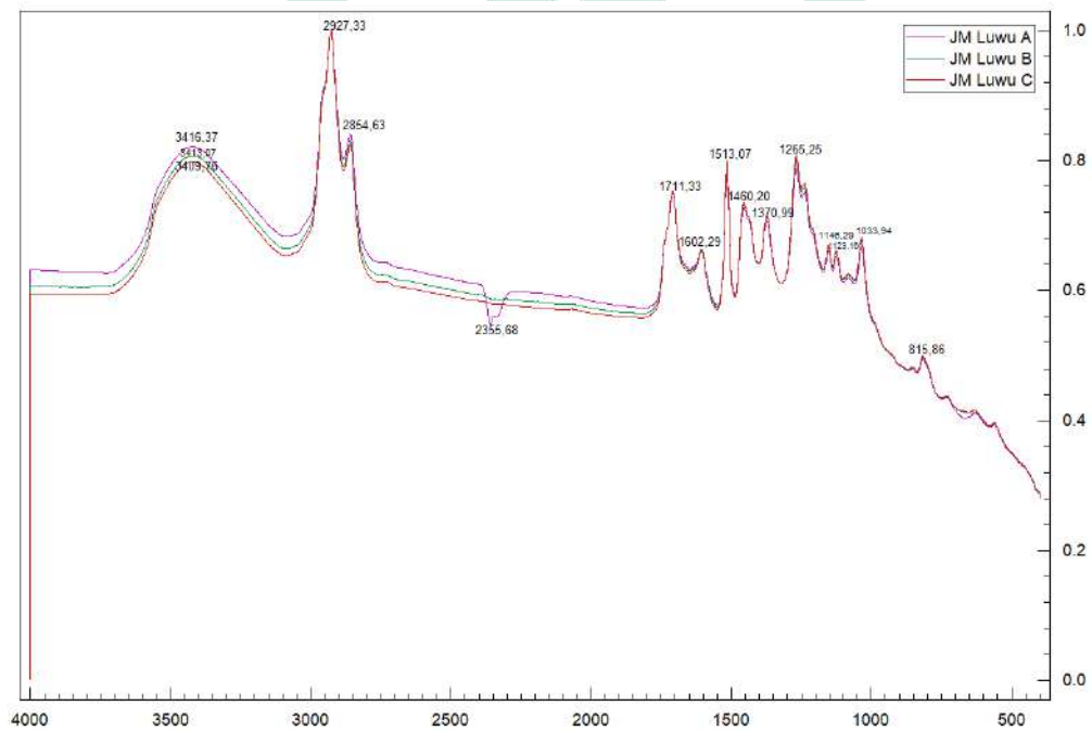
Gambar 4. 4. Spektrum Jahe Merah Luwu
