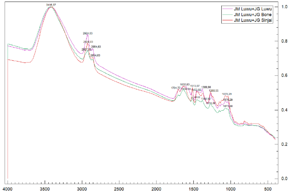
Gambar 4. 24. Spektrum Kombinasi Jahe Merah Luwu dan Jahe Gajah Bone, Jahe Gajah Luwu, dan Jahe Gajah Sinjai
