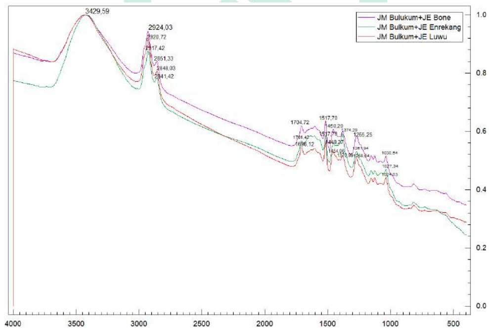
Gambar 4. 14. Spektrum Kombinasi Jahe Merah Bulukumba dan Jahe Emprit Enrekang, Jahe Emprit Bone, dan Jahe Emprit Luwu
