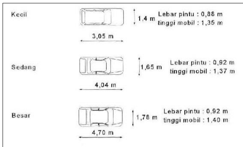
Gambar IV.2 Standar Dimensi Untuk Kendaraan Umum (Sumber : Juwono dan Victor, 1994)
