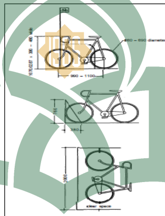
Gambar IV.4 Standar Dimensi Untuk Sepeda (Sumber : Planning and Design Data)
