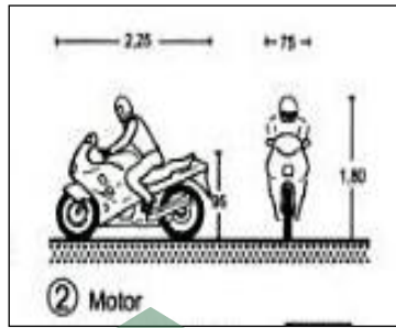
Gambar IV.3 Standar Dimensi Untuk Motor (Sumber : Data Arsitek Jilid 2)
