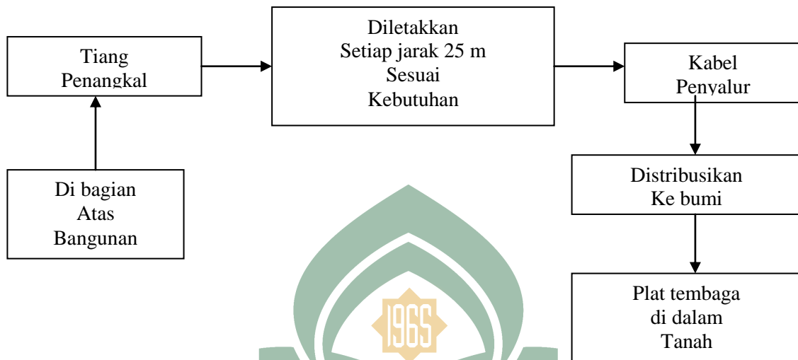
Gambar IV.18 Skema Sistem Penangkal Petir (Sumber : Sistem Bangunan Pintar, 2006)
