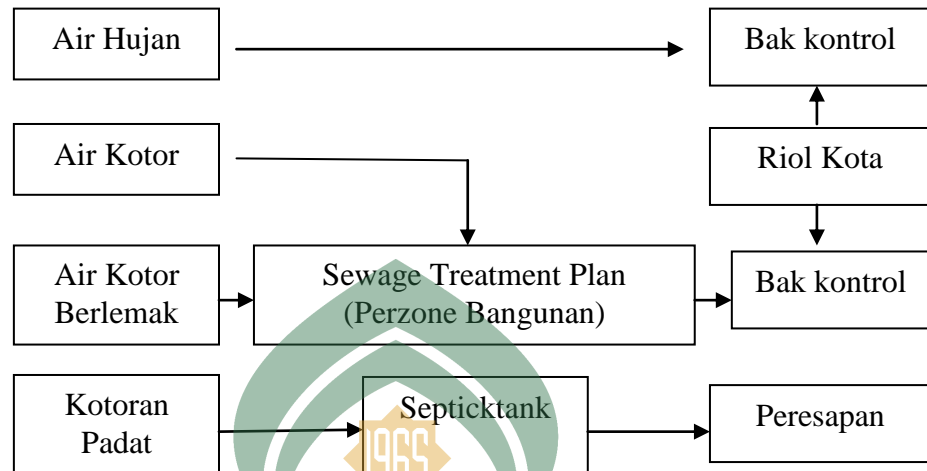
Gambar IV.15 Skema Sistem Pembuangan Air Kotor (Sumber : Sistem Bangunan Pintar, 2006)
