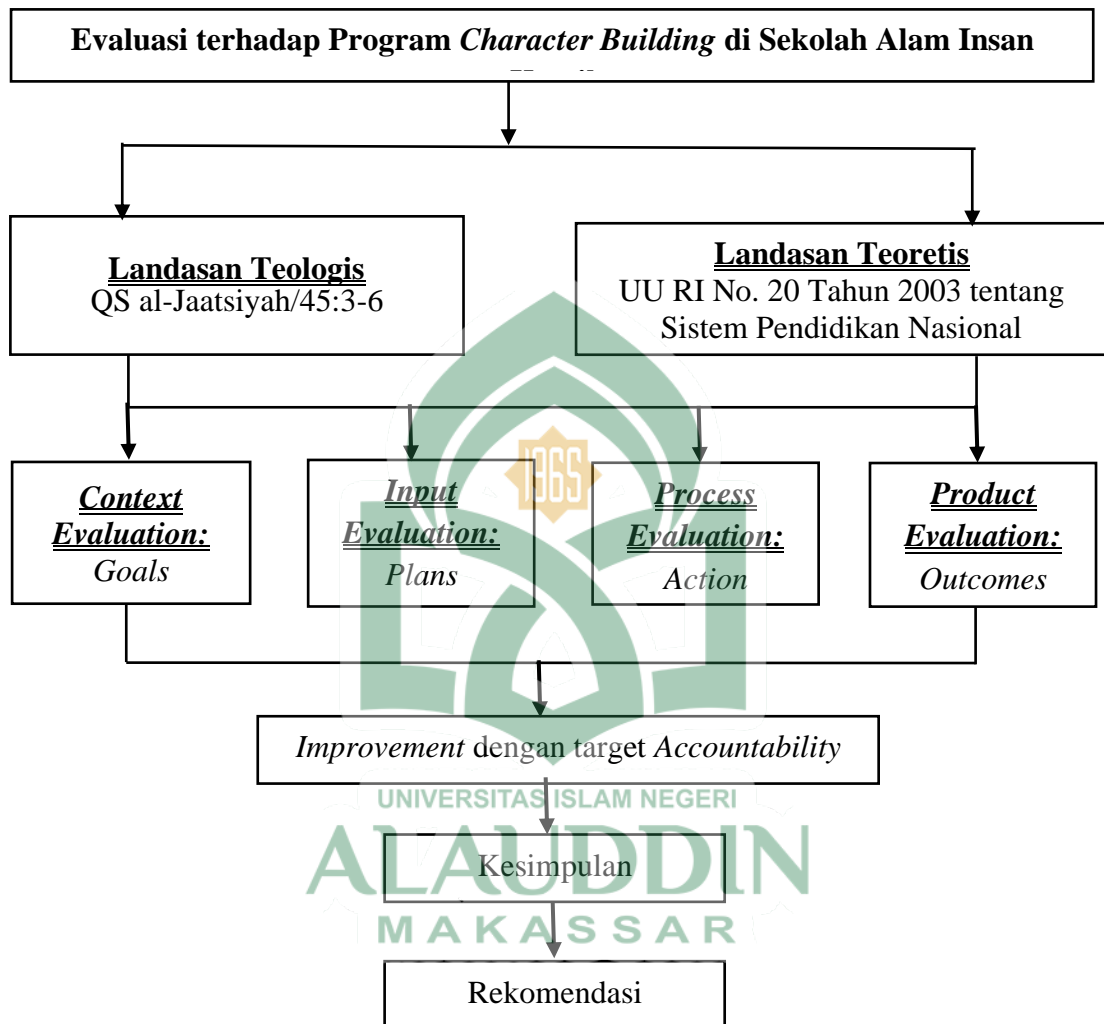
Gambar 2.1 Kerangka Konseptual
