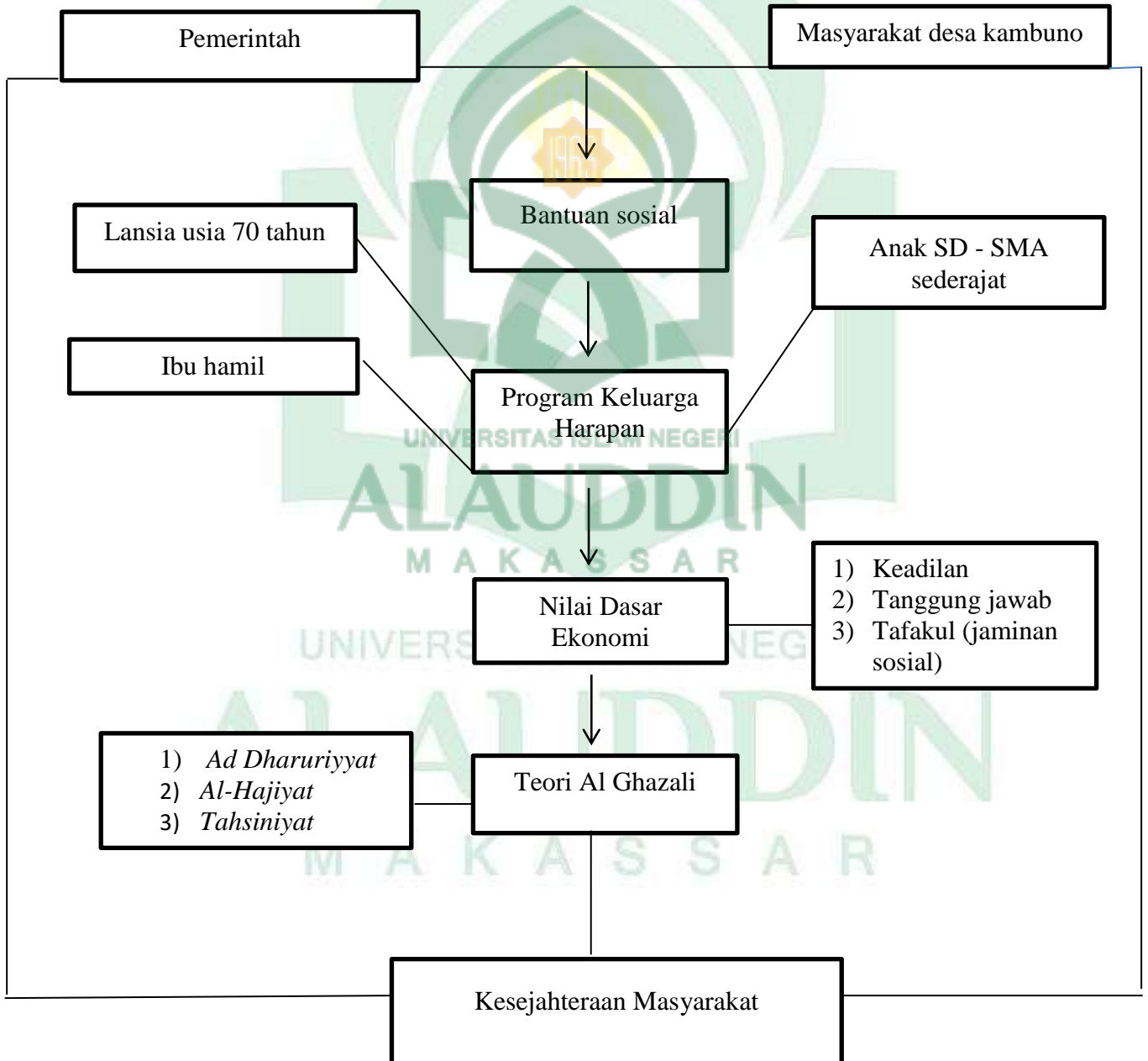
gambar 2.1 kerangka pikir
