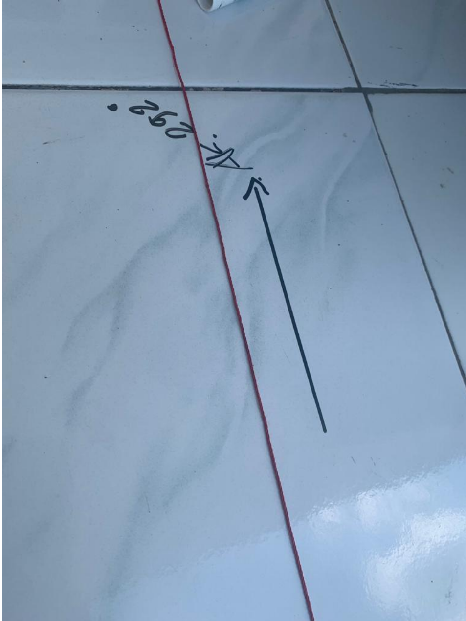
PENGUKURAN ARAH KIBLAT MASJID SULTAN ALAUDDIN MADANI MENGUNAKAN TONGKAT ISTIWA'
