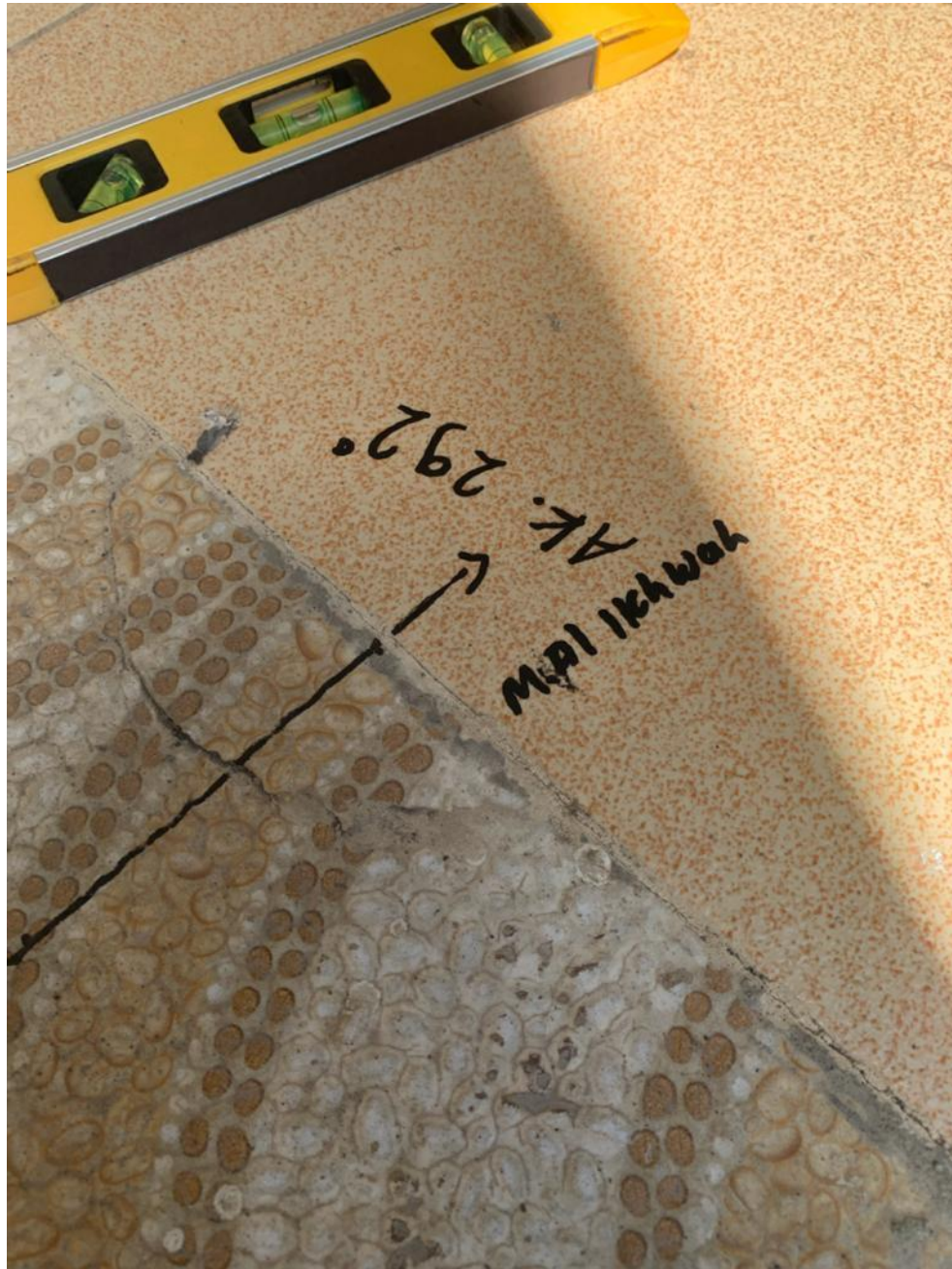
PENGUKURAN ARAH KIBLAT MASJID NURUL IKHWAH MENGUNAKAN TONGKAT ISTIWA'
