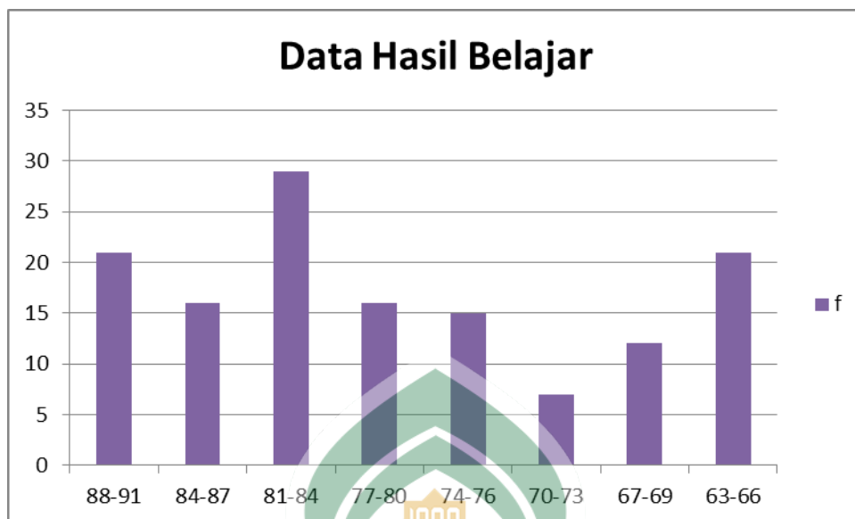
Gambar 1.3. histogram hasil belajar kognitif
