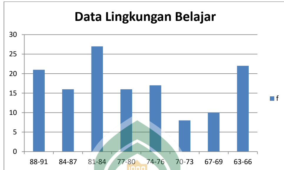
Gambar 1.2 Histogram lingkungan belajar
