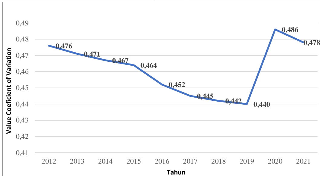
Gambar 4.6 Konvergensi Sigma
