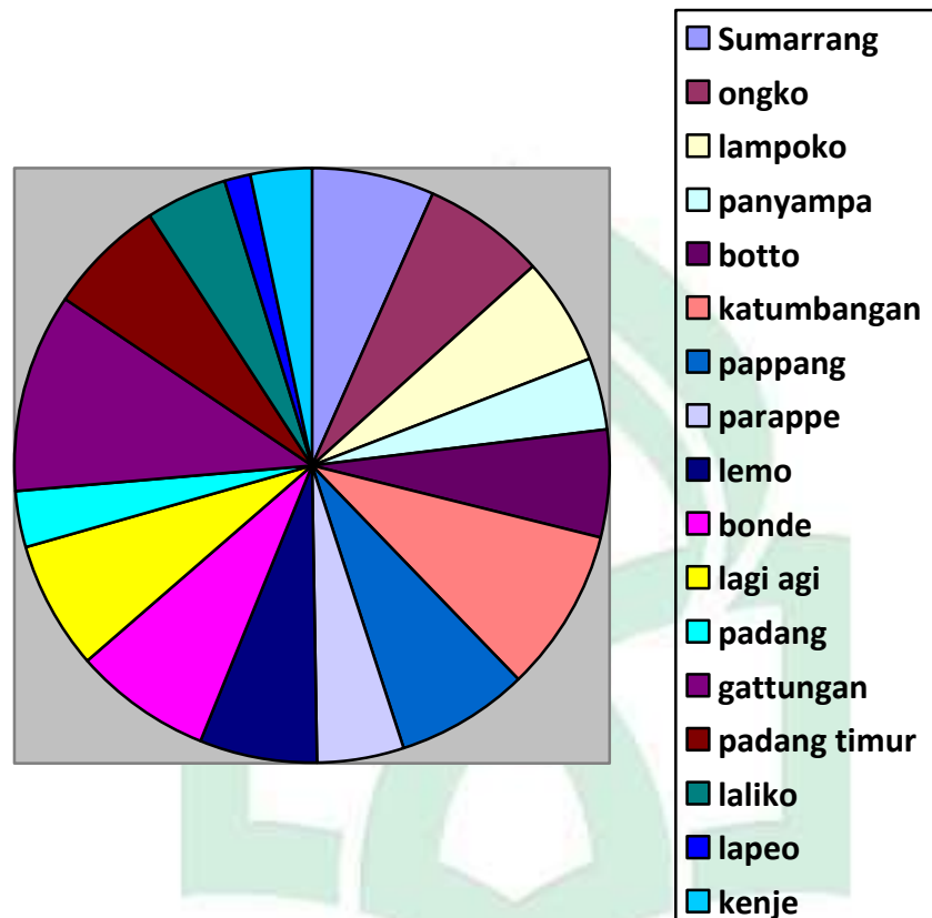
Grafik 1 Luas Wilayah Desa / Kelurahan Di Kecamatan Campalagian
