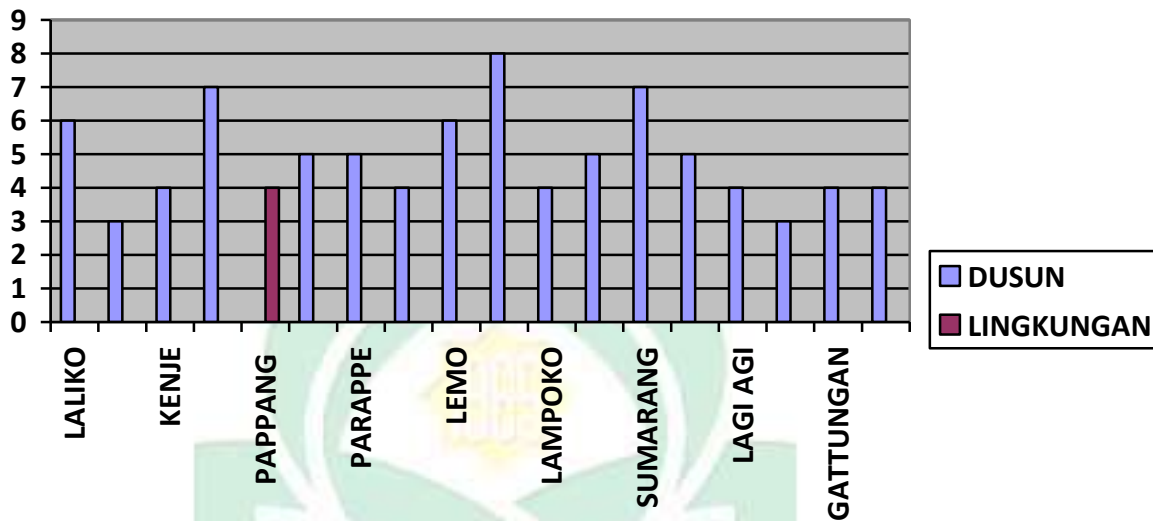
Grafik 2 Jumlah Dusun/Lingkungan Menurut Desa/Kelurahan di Kecamatan Campalagian
