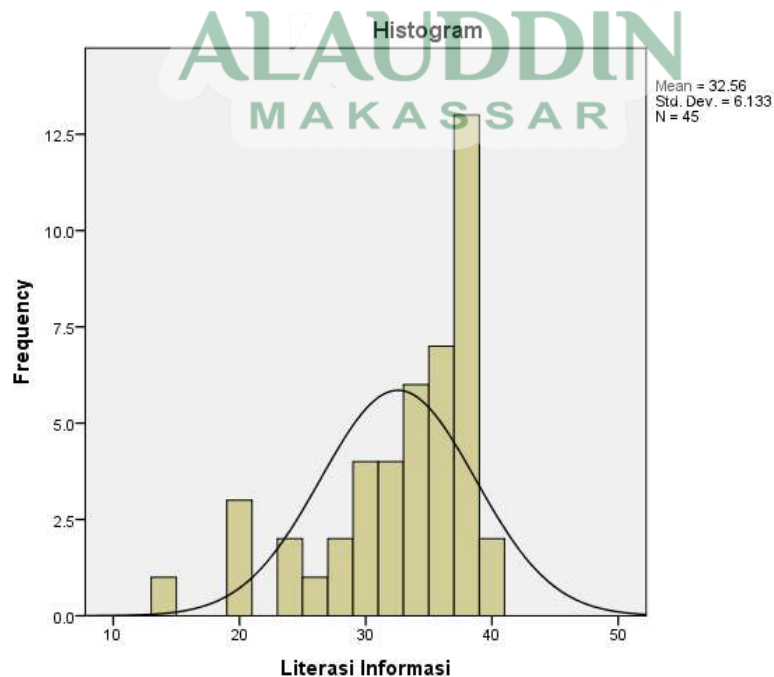
4.1 Gambar Histogram Literasi Informasi (X 1 )
