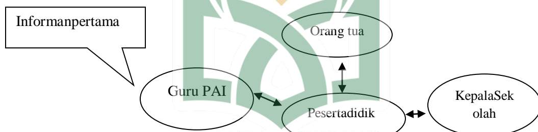
Gambar 2 Triangulasi Sumber
