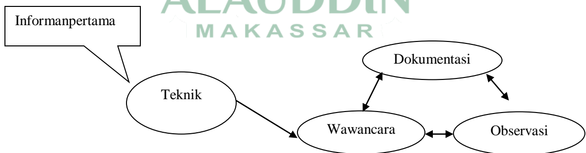
Gambar 3 Triangulasi Teknik
