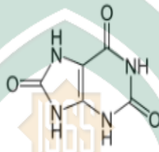
Gambar 2. Rumus bangun asam urat : C_5H_4N_4O_3 (Ganong, 2008).
