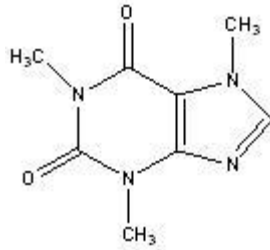
Gambar 6. Struktur kafeina
