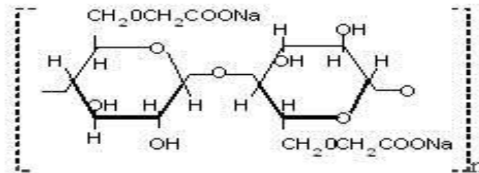
Gambar 7. Struktur Na-CMC
